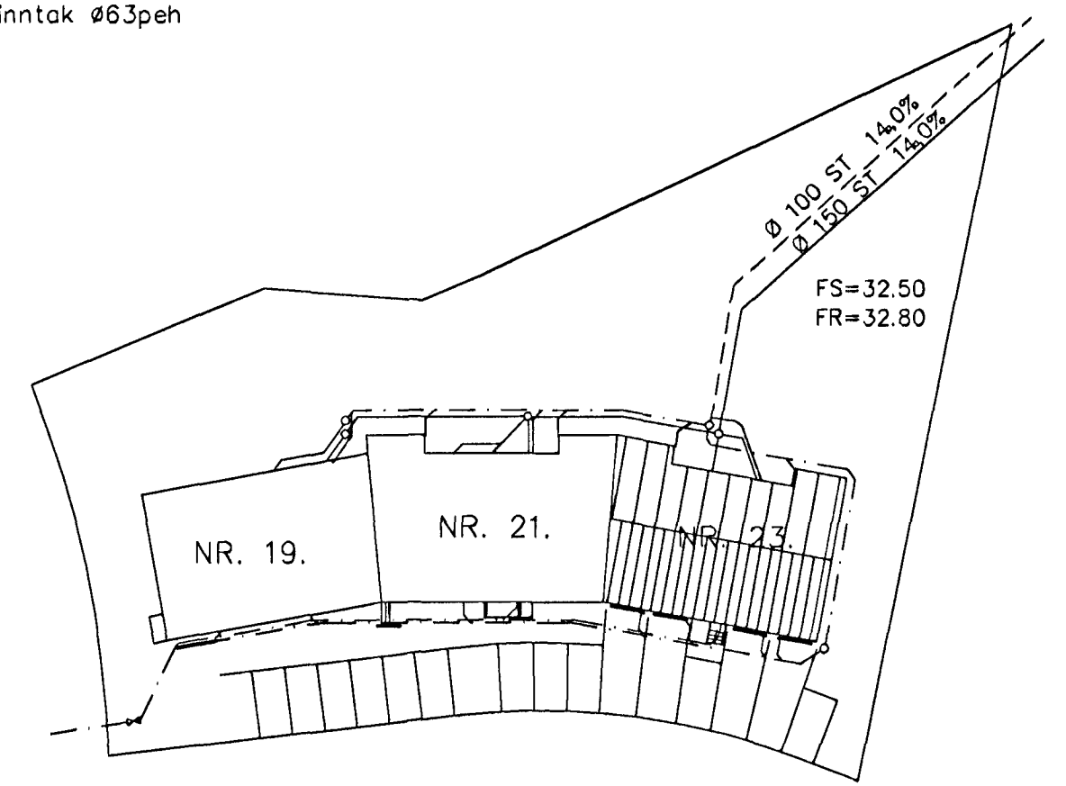
AFSTÖÐUMYND 1:500
