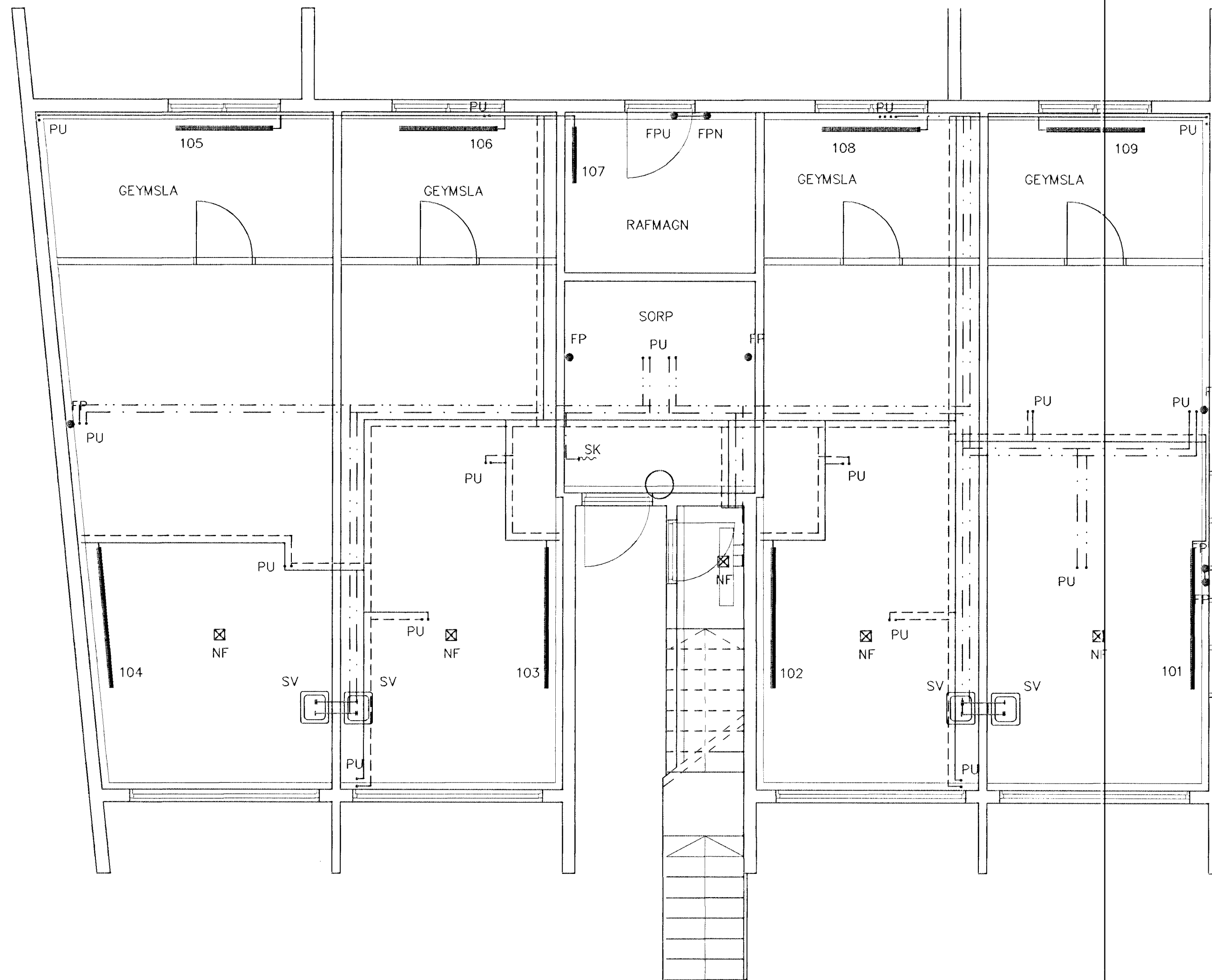
GRUNNMYND 1 HÆÐAR 1:50
