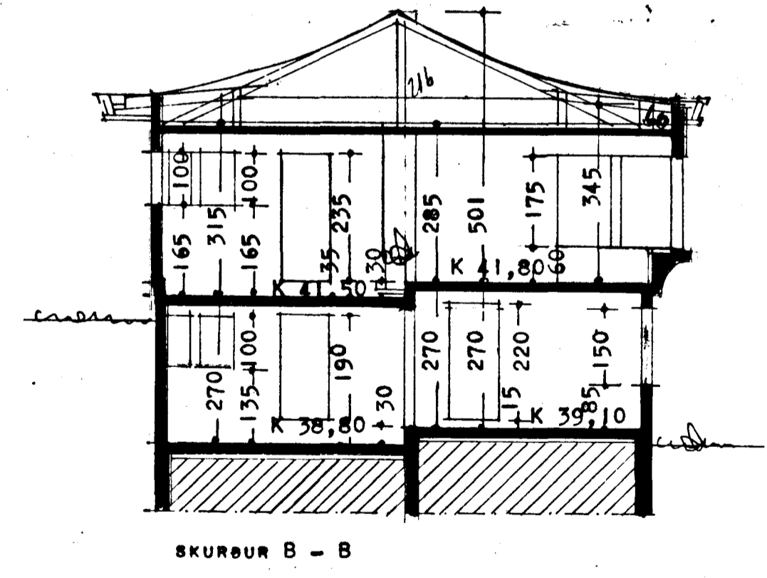
ANNARS SKV. SÉRUPPDRÁTTUR F M 1:20
