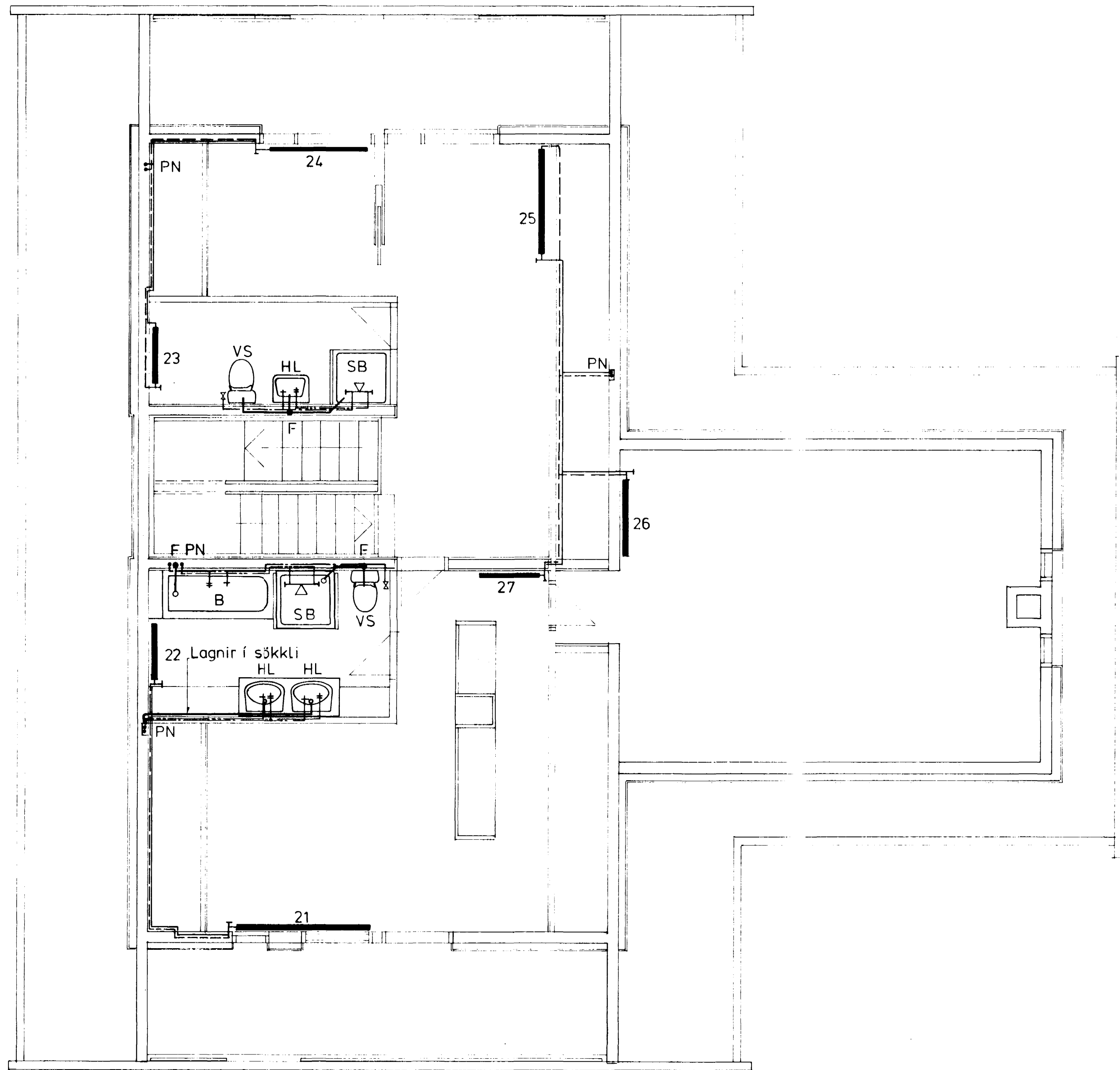
GRUNNMYND 2.HÆÐAR 1:50
