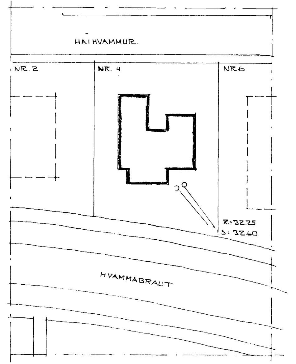
AFSTÖÐUMYND 1:500
