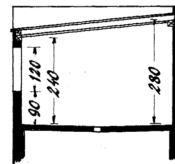
Þverskurður
