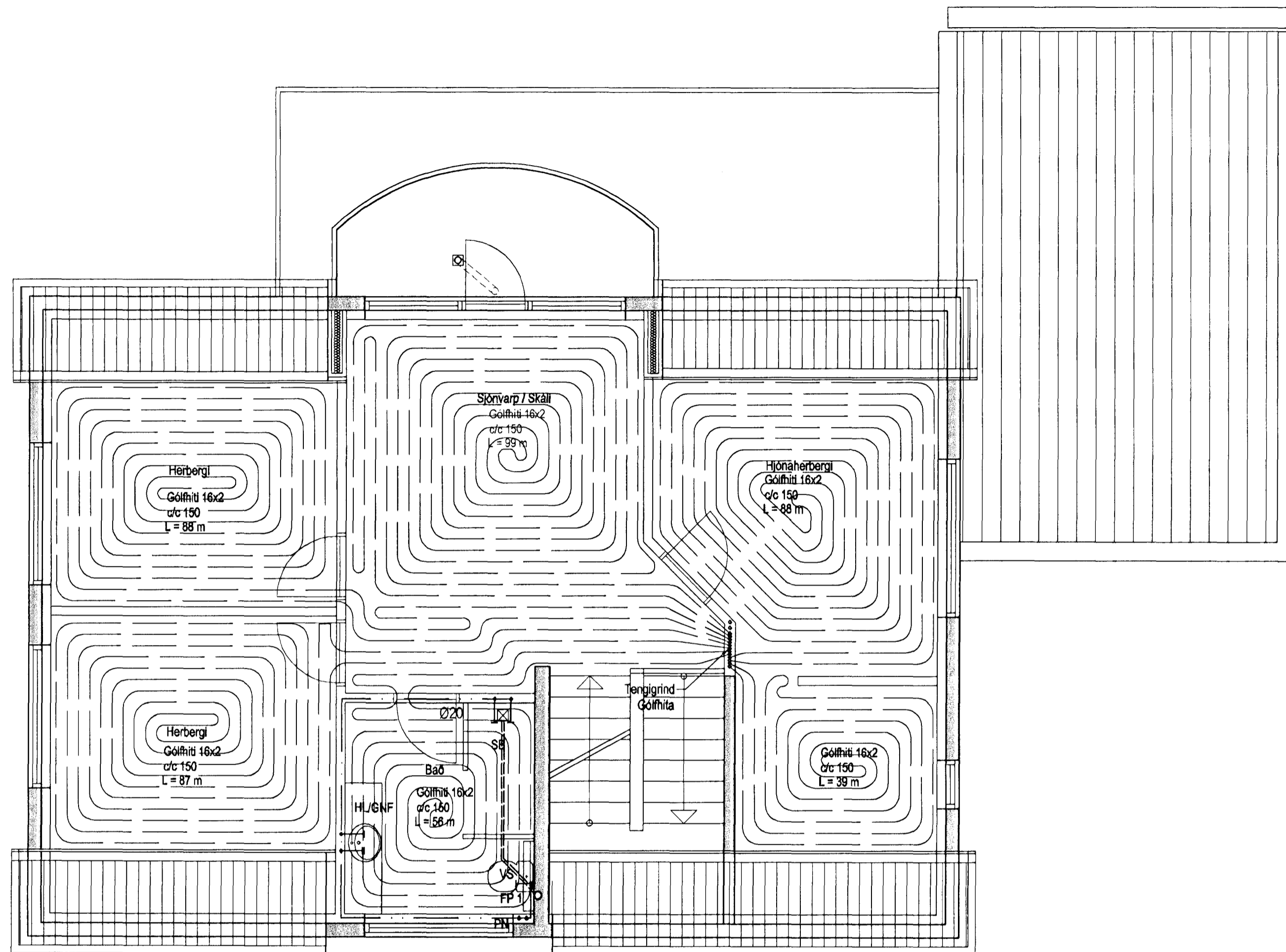
3. hæð, Gólfhitalagnir, Grunnmynd, 1:50
