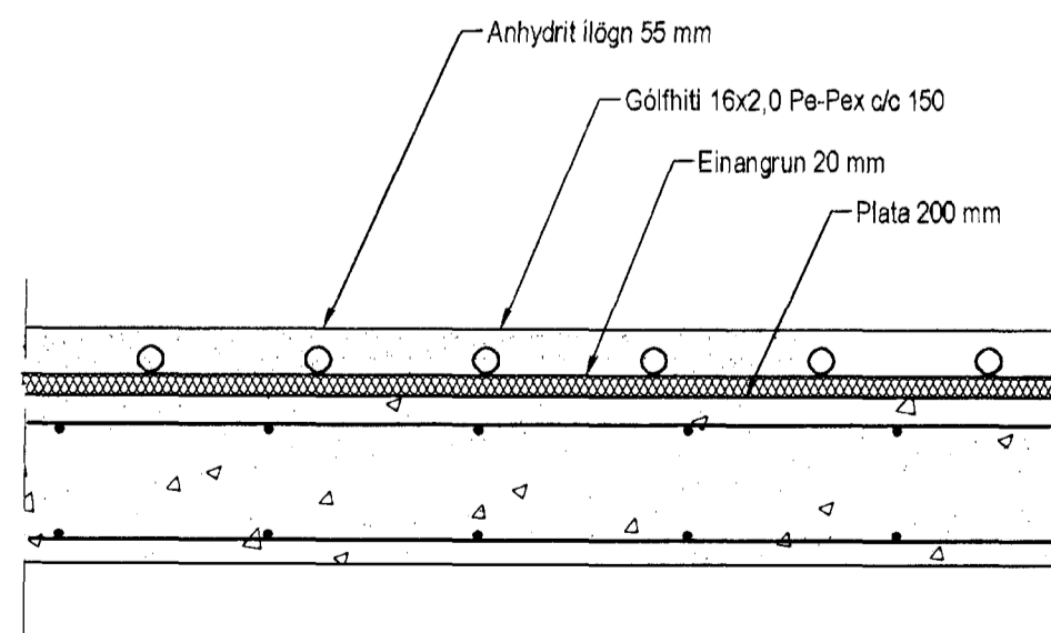
Hita- og vatnslagnir, Snið í milliþötu, 1:10
