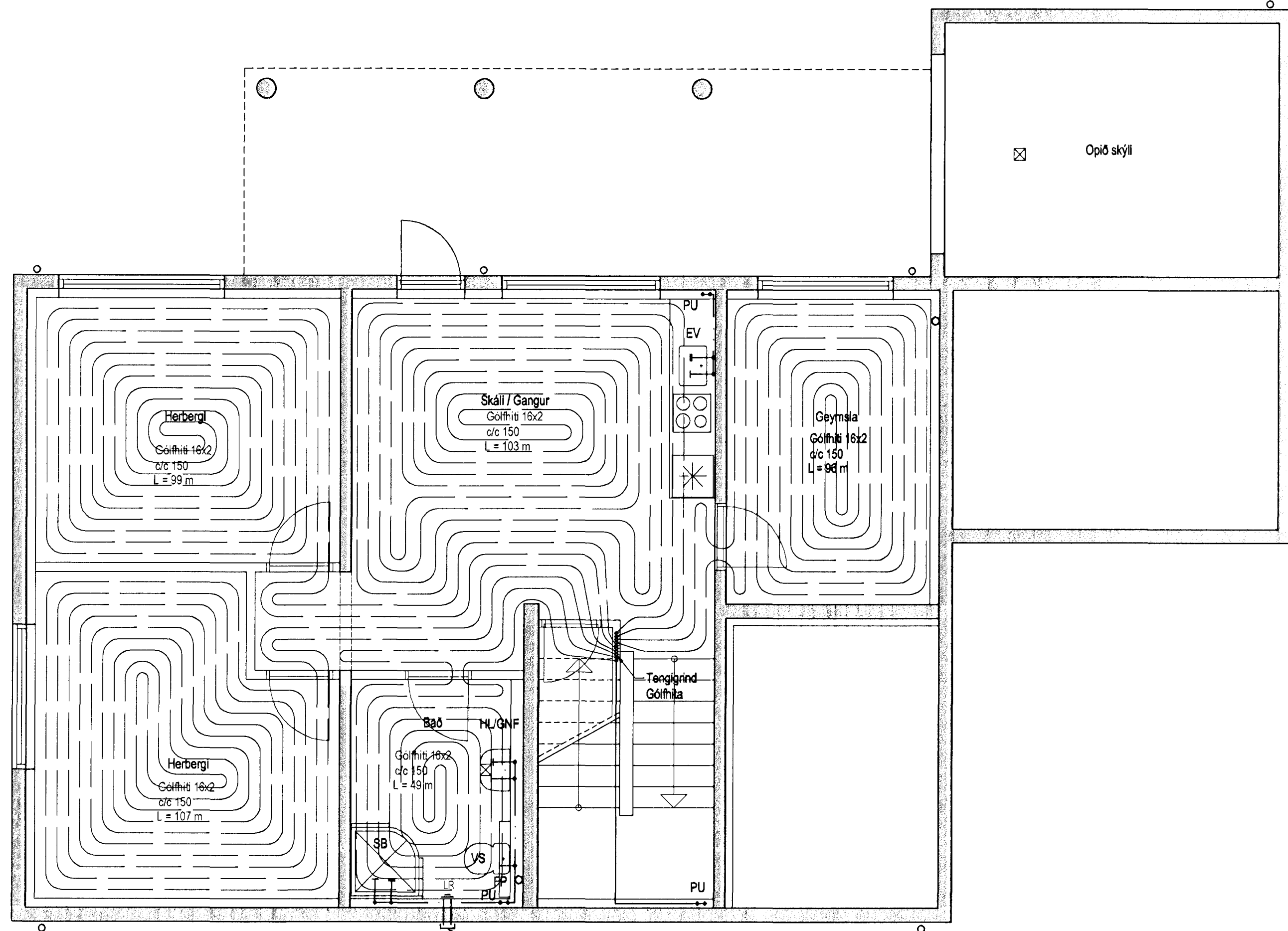
1. hæð, Gólfhitalagnir, Grunnmynd, 1:50
