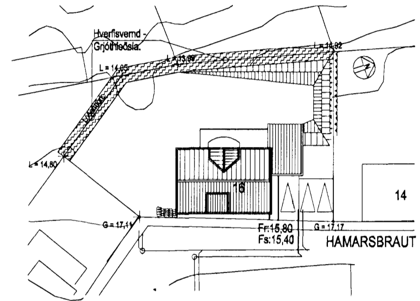
Afstöðumynd 1:500
