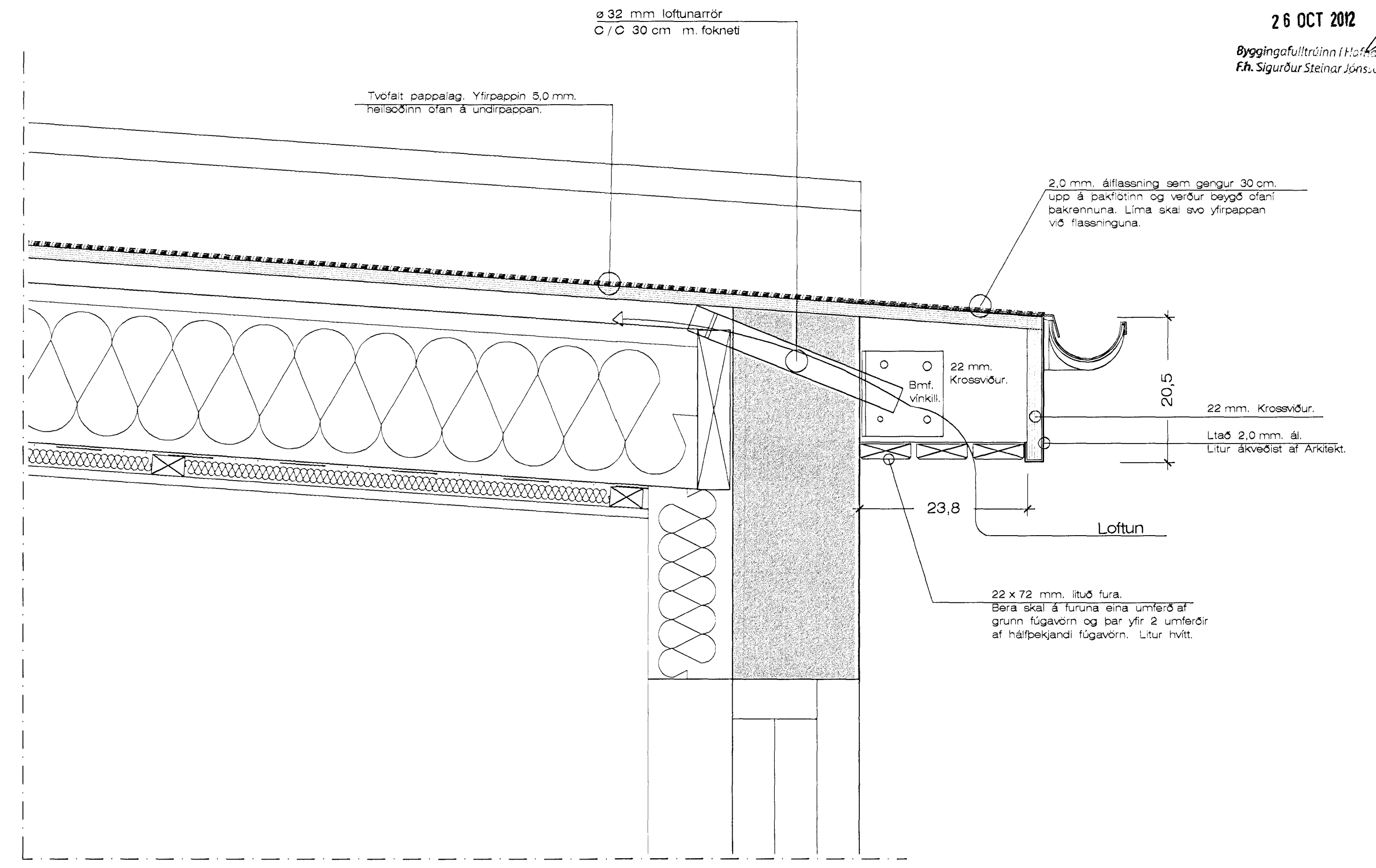
Þakkantur á bílgeymslu. 1 : 5
