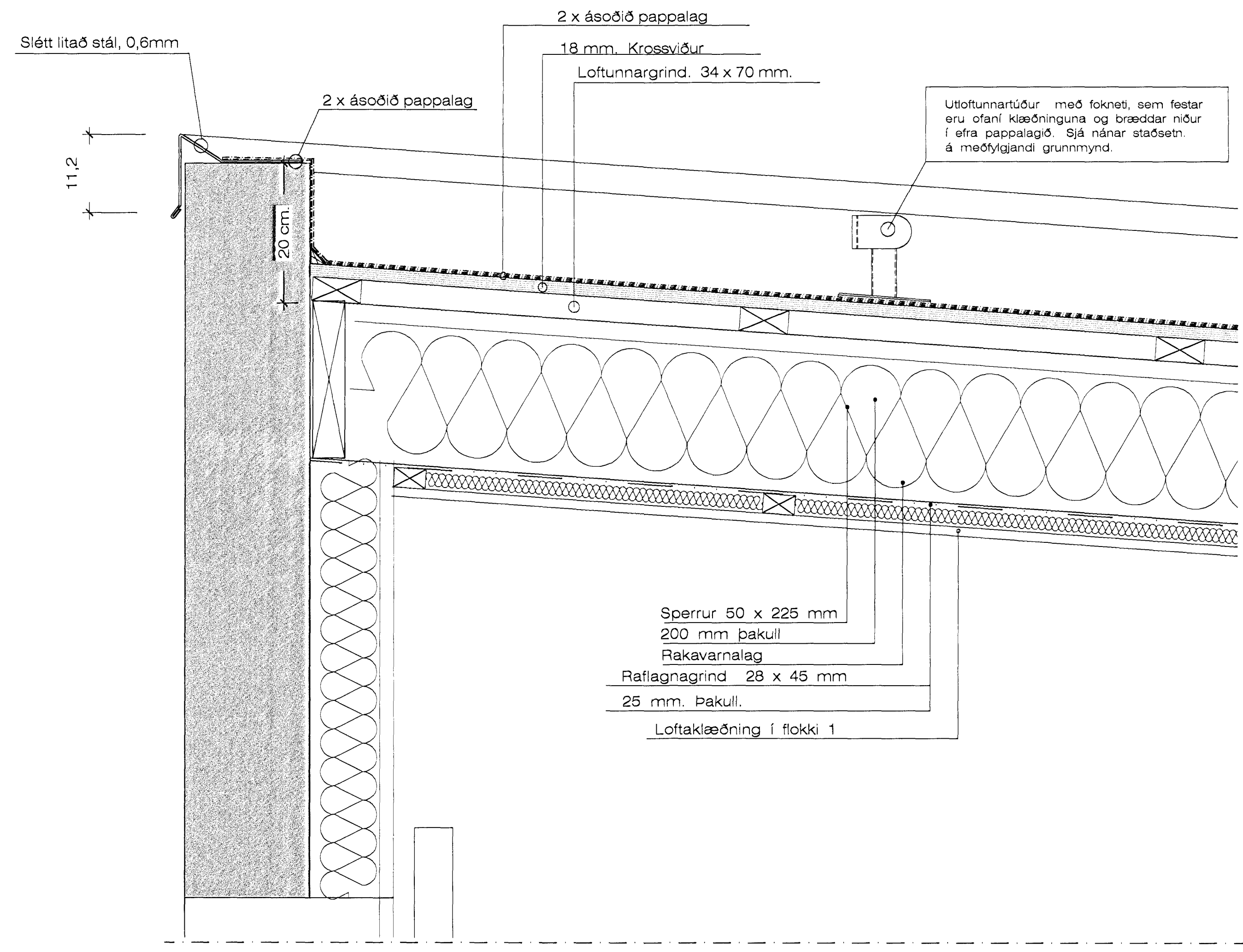
Þakkantur á bílgeymslu. 1 : 5
