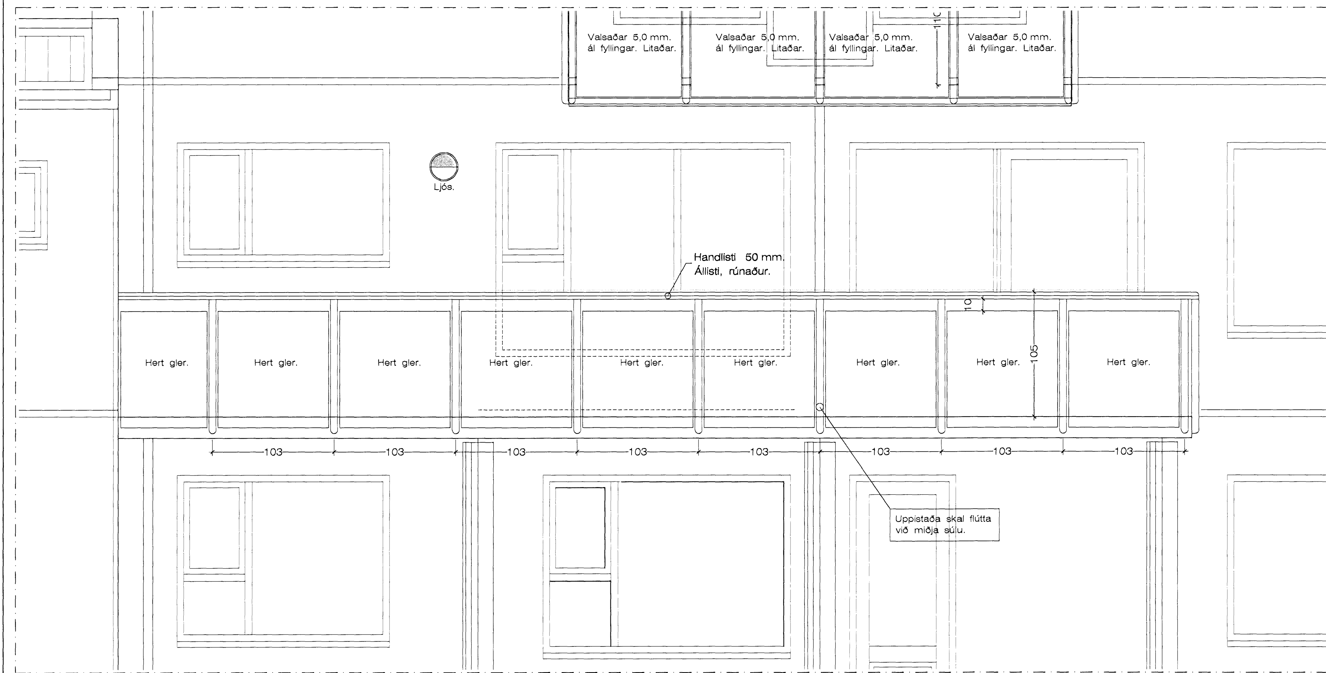
Séð framaná svalahandrið. Á 1. hæð. 1 : 20
