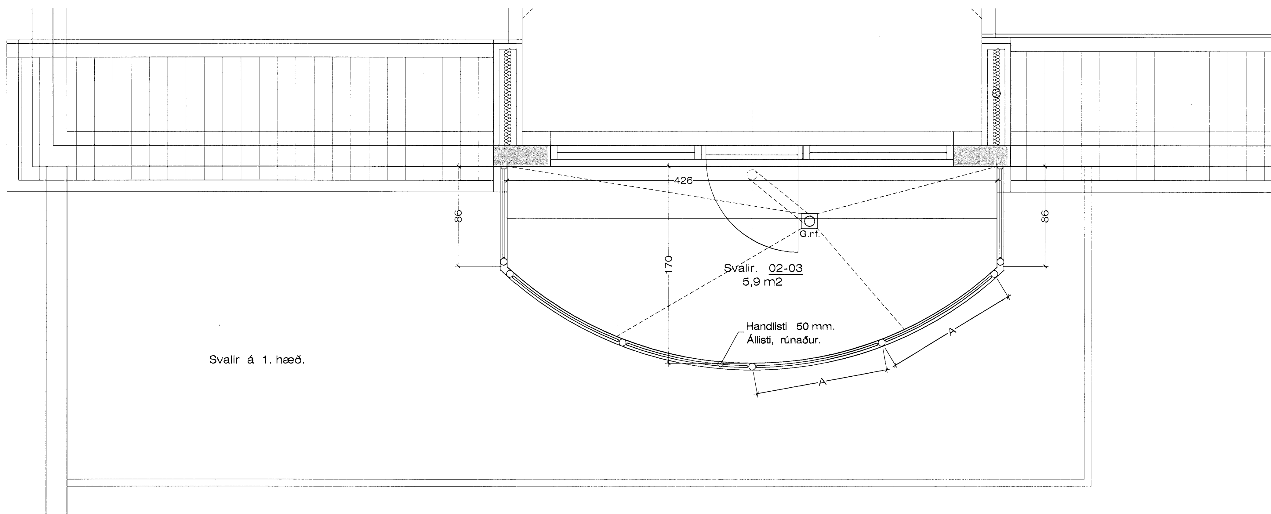
Grunnmynd af svalahandriði. 1 : 20
