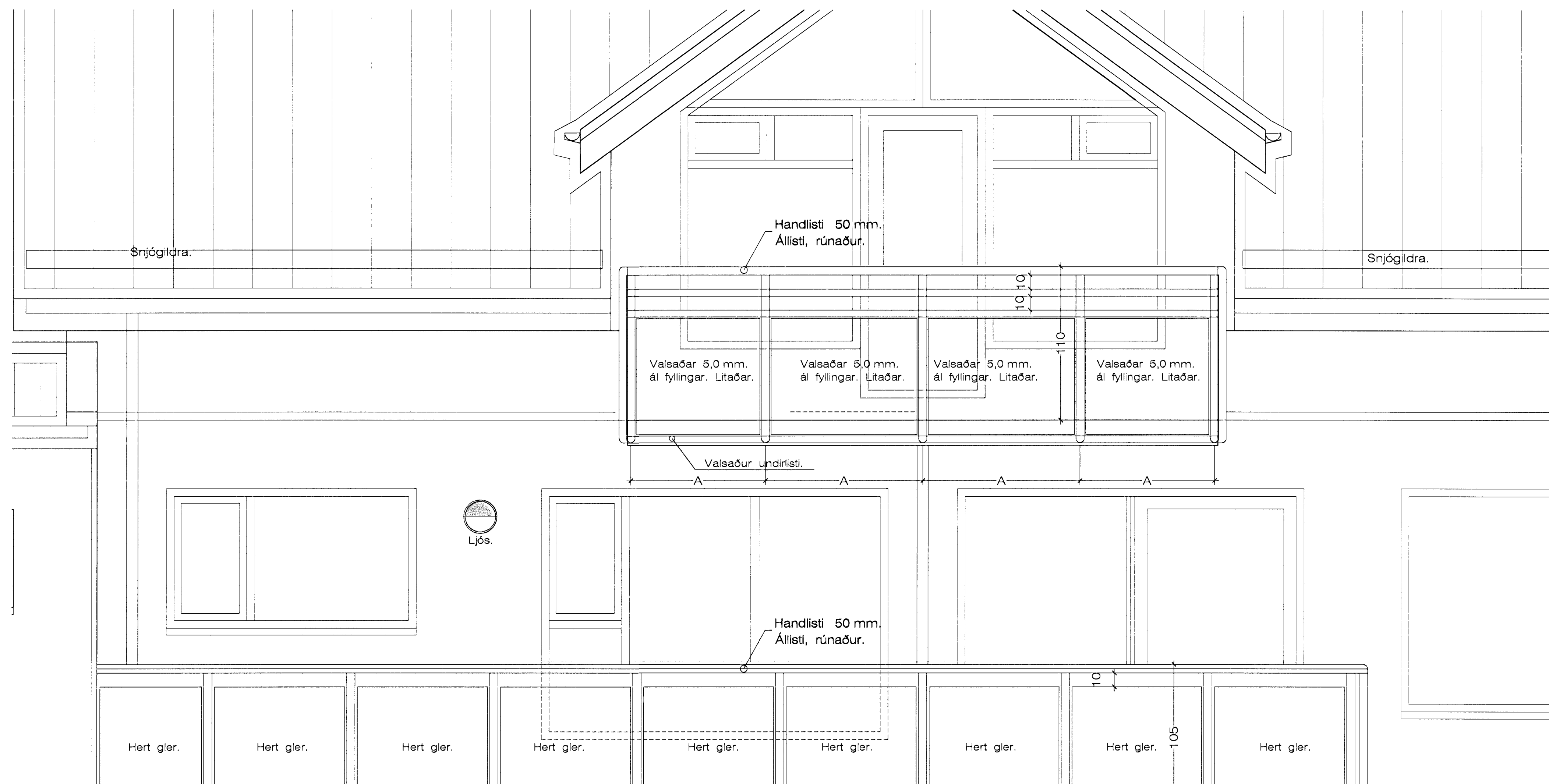
Séð framaná svalahandrið. Á 2. hæð. 1 : 20
