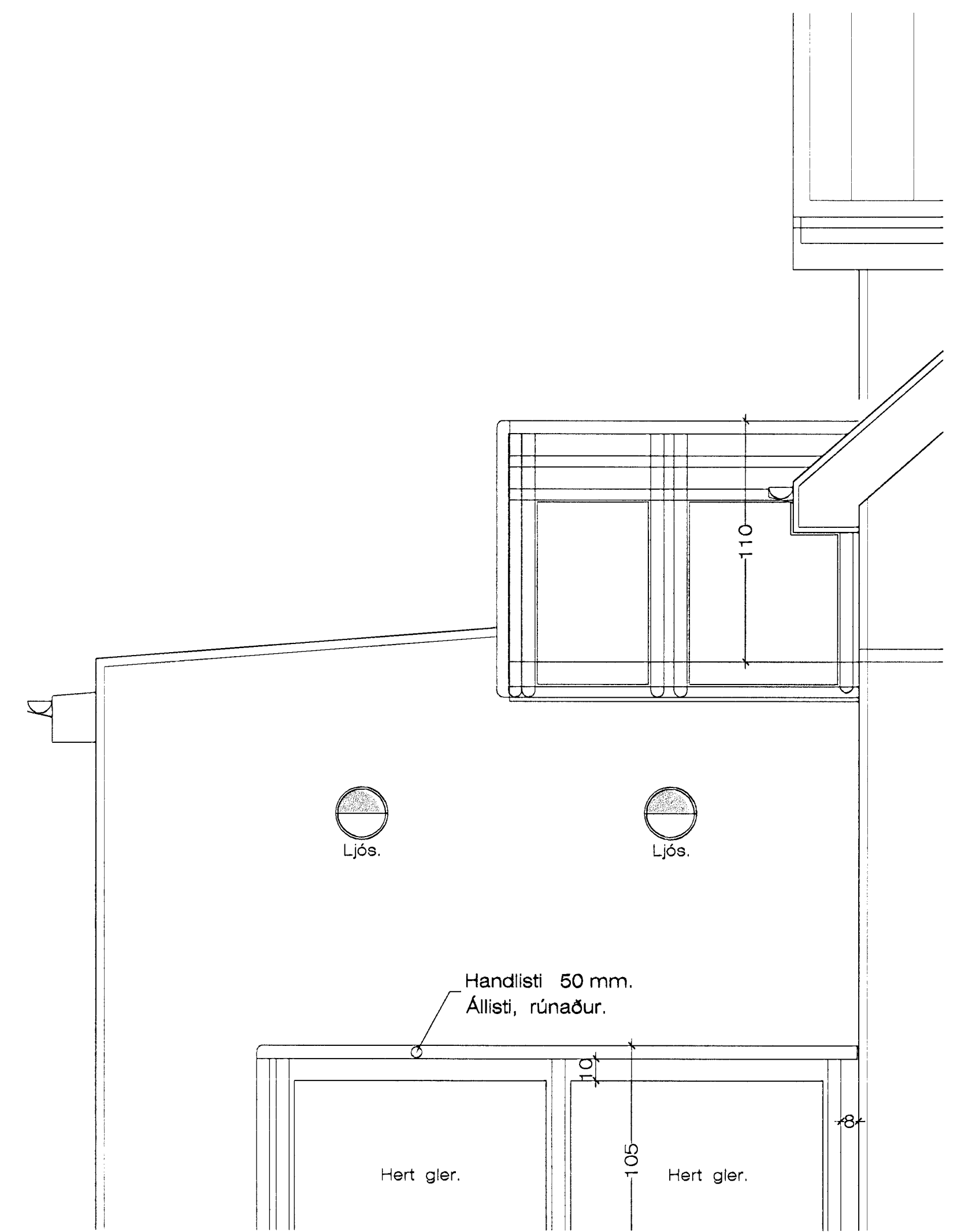
Hliðarmynd af svalahandrið. Á 1. hæð. 1 : 20
