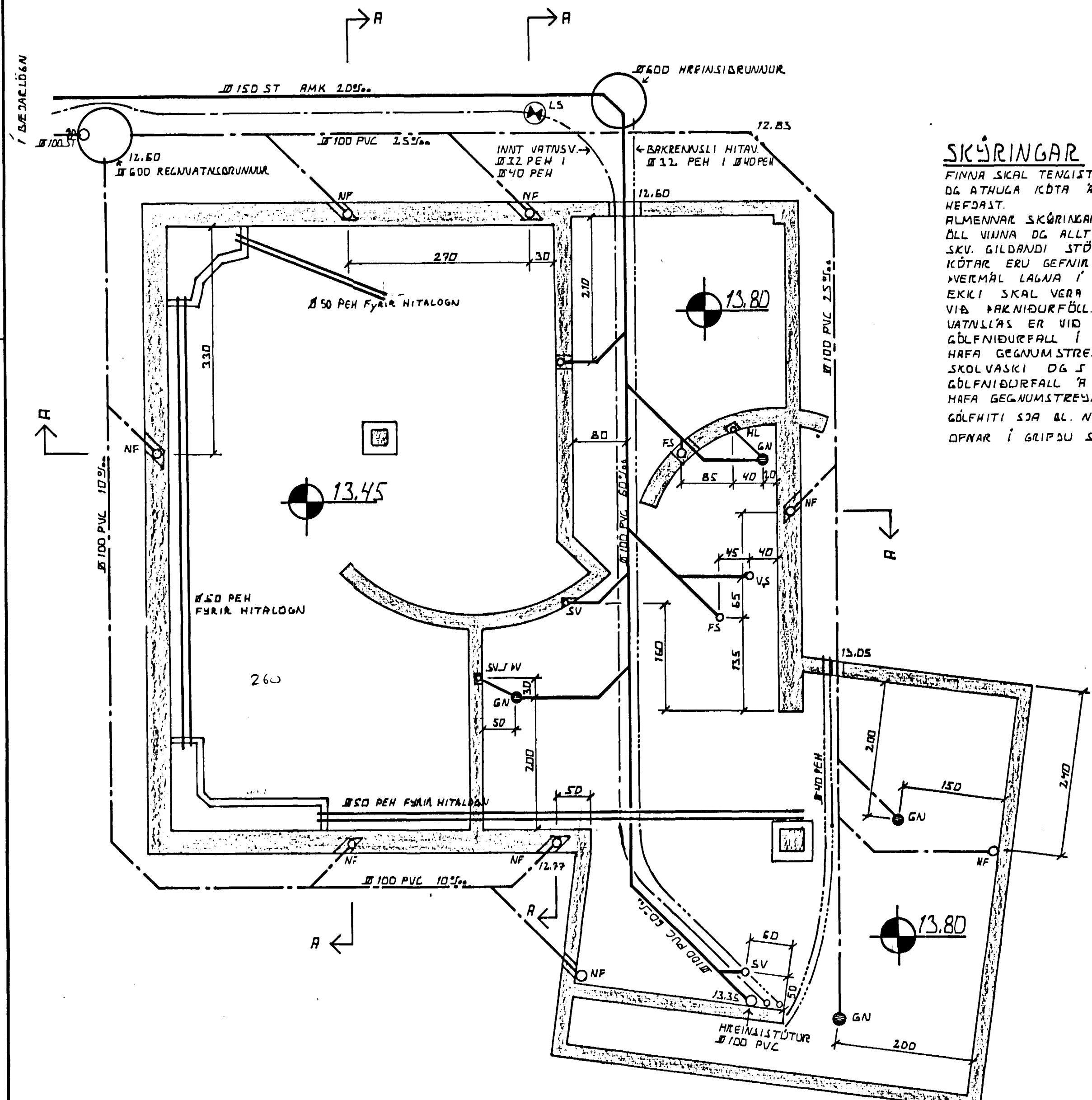
GRUNNMYND 1:50
