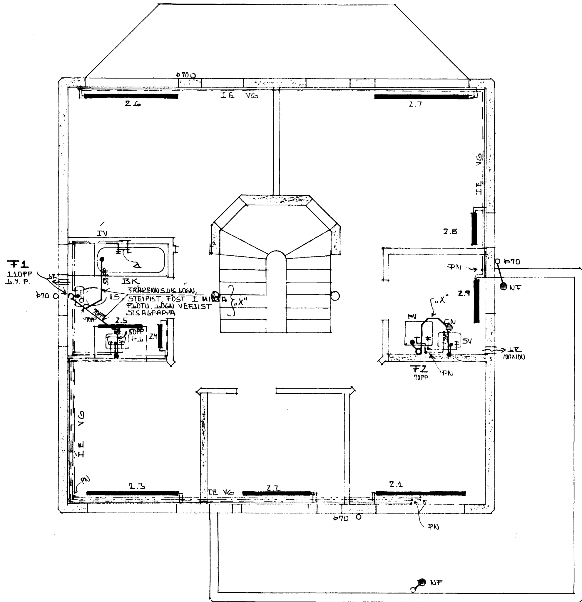
GRUNNMYND 1:50
