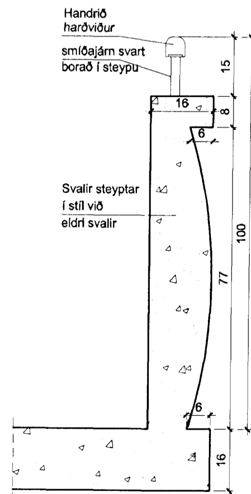
Handrið svalir - Mkv 1:5
