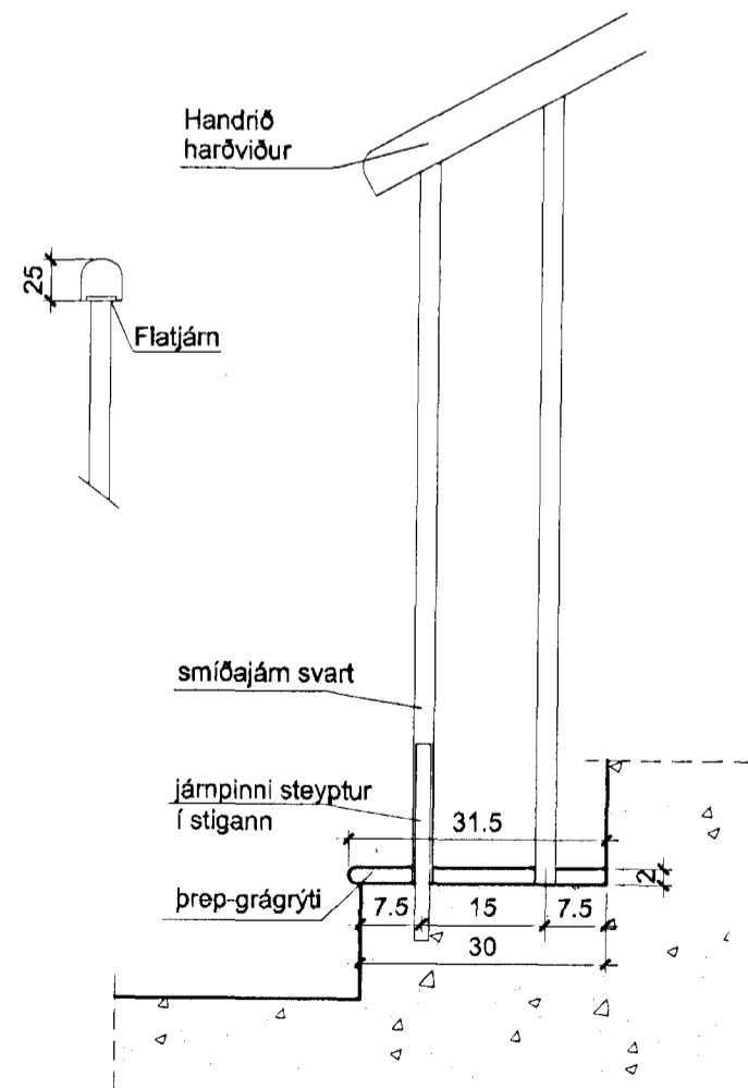
Handrið stigi - Mkv 1:5
