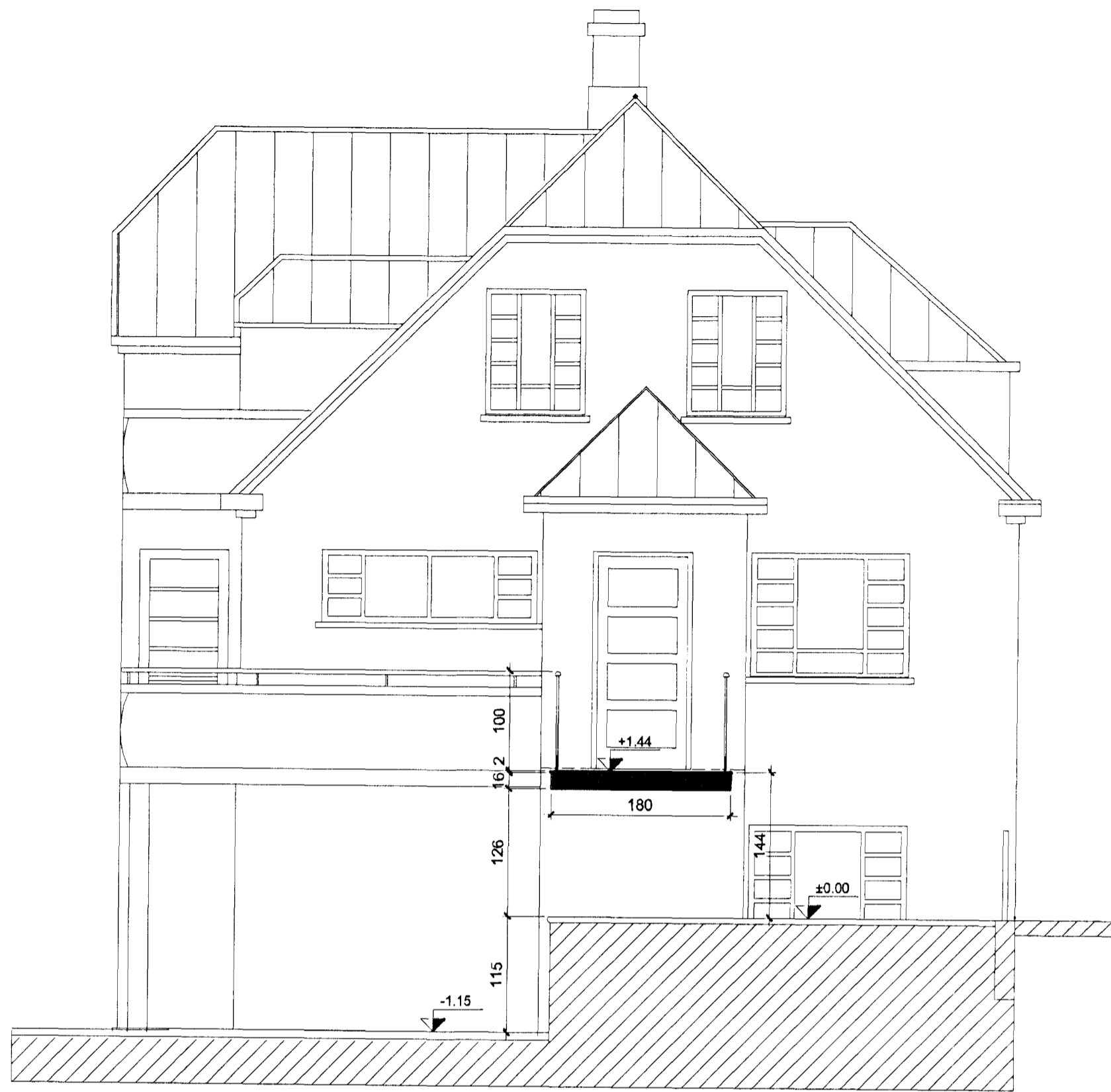
Snið C-C
