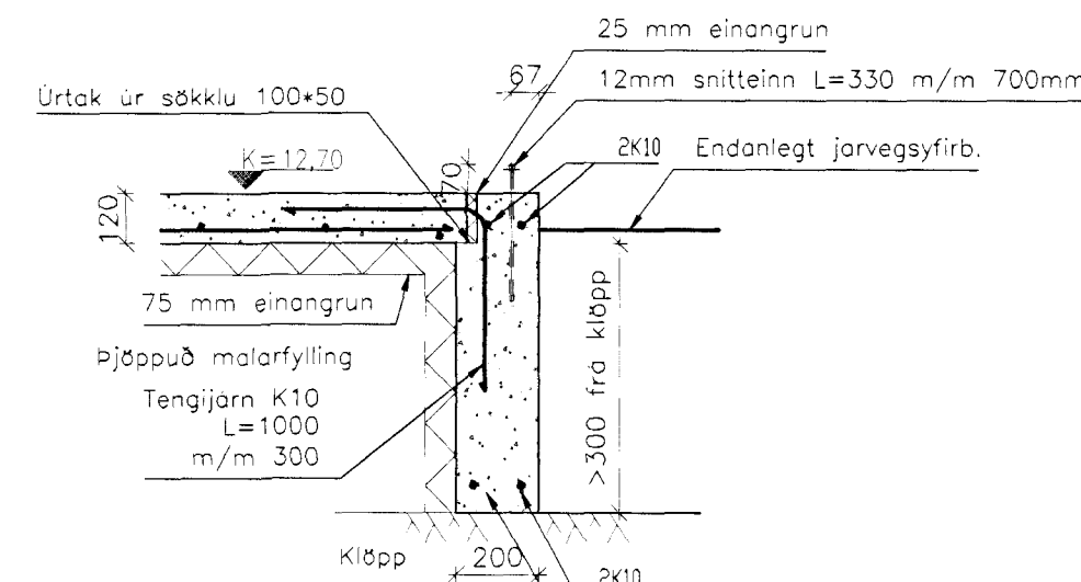
1 SKURÐUR Í SÖKKULÚTVEGG Mkv: 1/20
