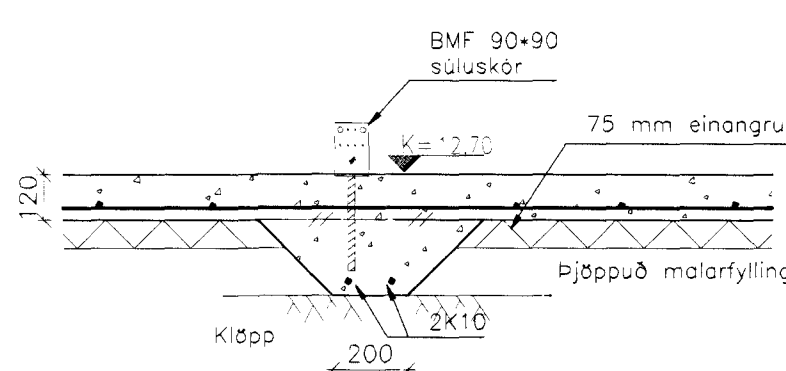
3 SKURÐUR VIÐ SÚLUFÖT Í MILLIVEGG Mkv: 1/20
