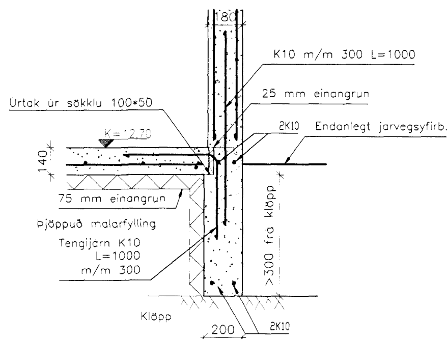
2 SKURÐUR Í SÖKKULÚTVEGG BILGEYMSLU Mkv: 1/20
