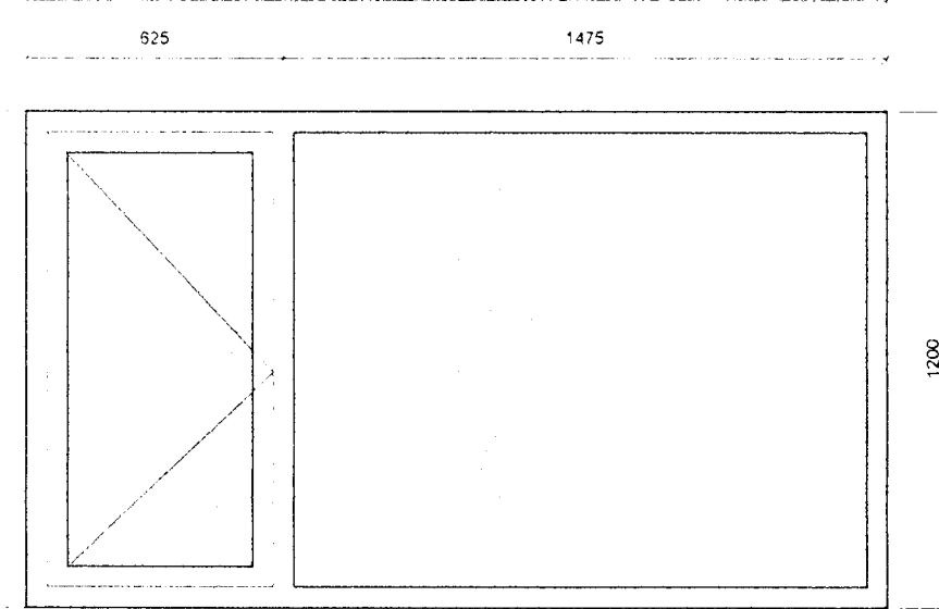
G-3, 1 stk. Efri brún 2150 mm yfir gólf Settur saman við G-2 samkvæmt deili 1.
