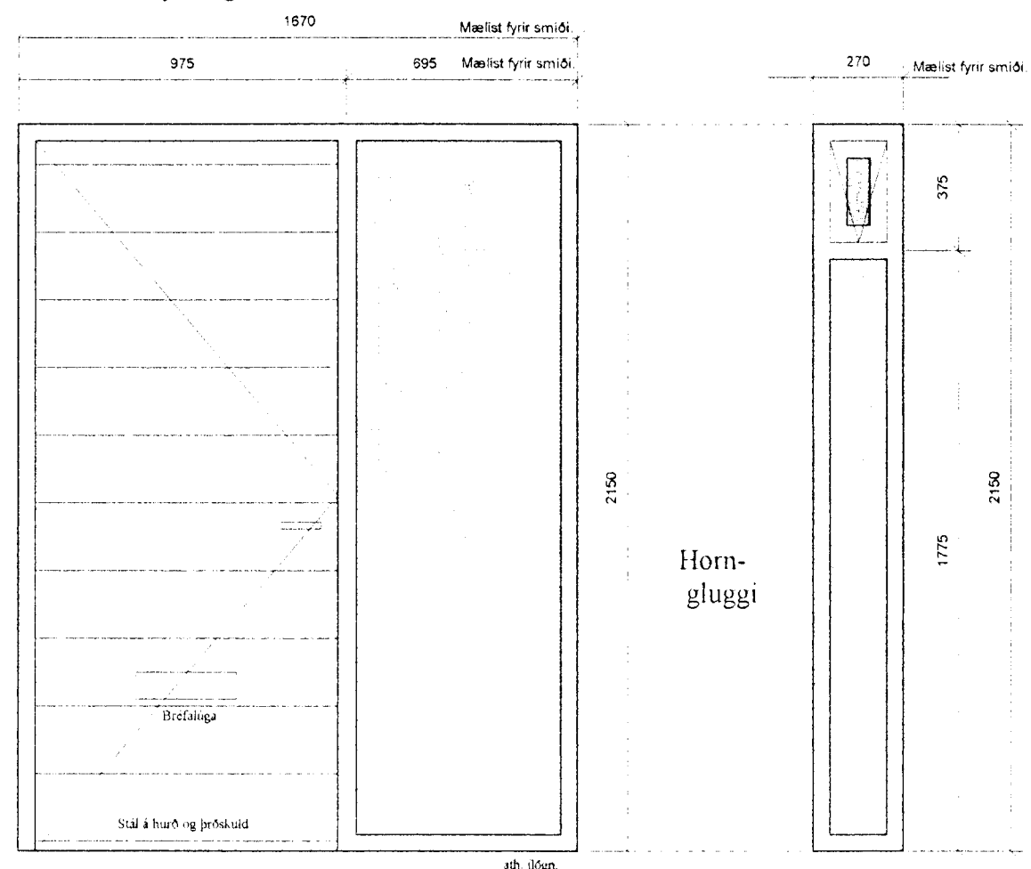
GH-1, 1 stk. Efri brún 2150 mm yfir gólf Mögulega sandblásið gler. Settur saman við G-10 samkvæmt deili 3.
