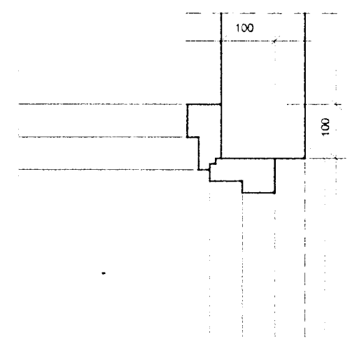
Deili 3, mkv. 1:10, Samsetning glugga G-10 við GH-1
