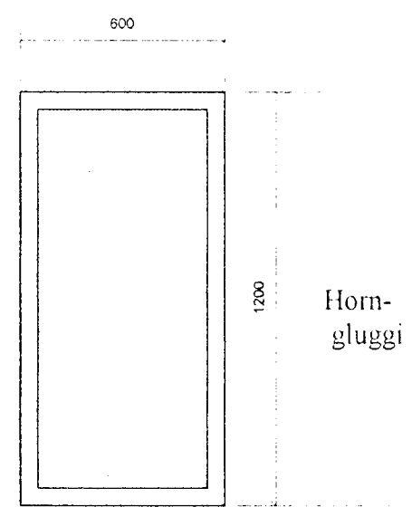
G-2, 1 stk. Efri brún 2150 mm yfir gólf Settur saman við G-3 samkvæmt deili 1.
