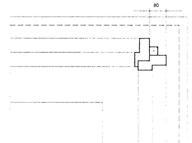
Deili 1, mkv. 1:10, Samsetning glugga G-2 við G-3 og einnig G-8 við G-9
