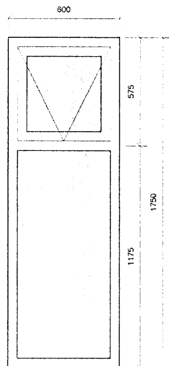
G-9, 1 stk. Efri brún 2150 mm yfir gólf Settur saman við G-8 samkvæmt deili 1.
