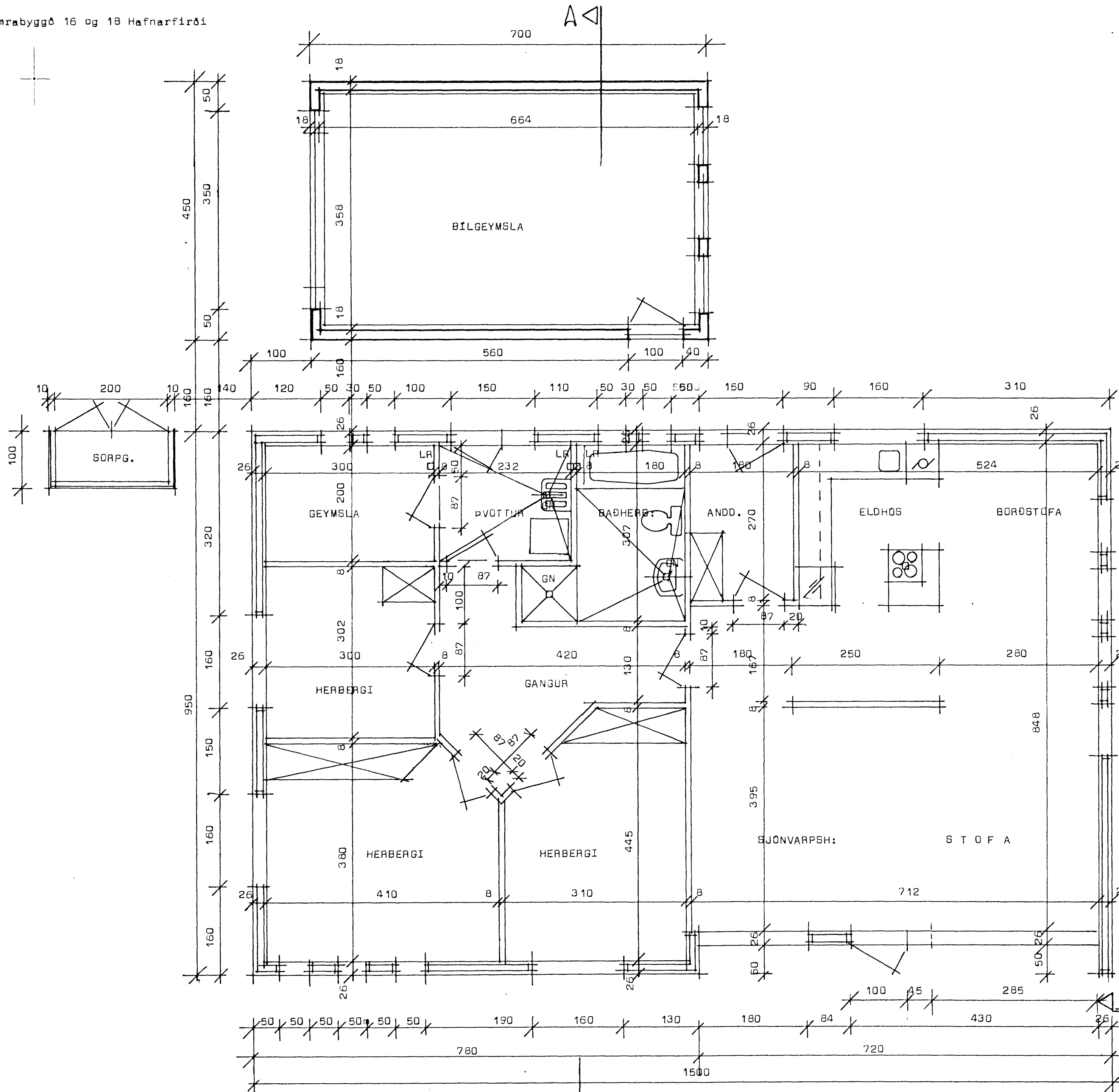
Grunnmynd MK 1:50
