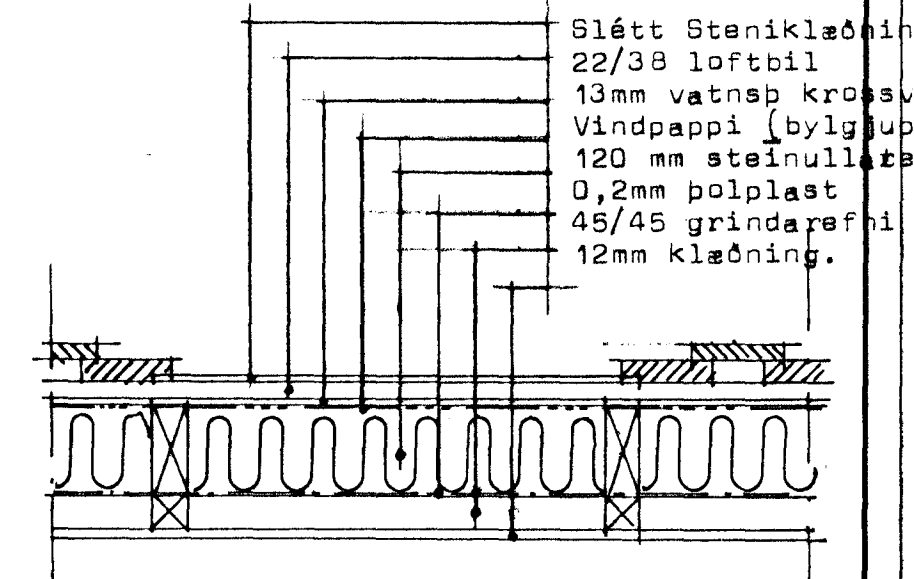
Lárétt snip undir og yfir glugga MK 1:20
