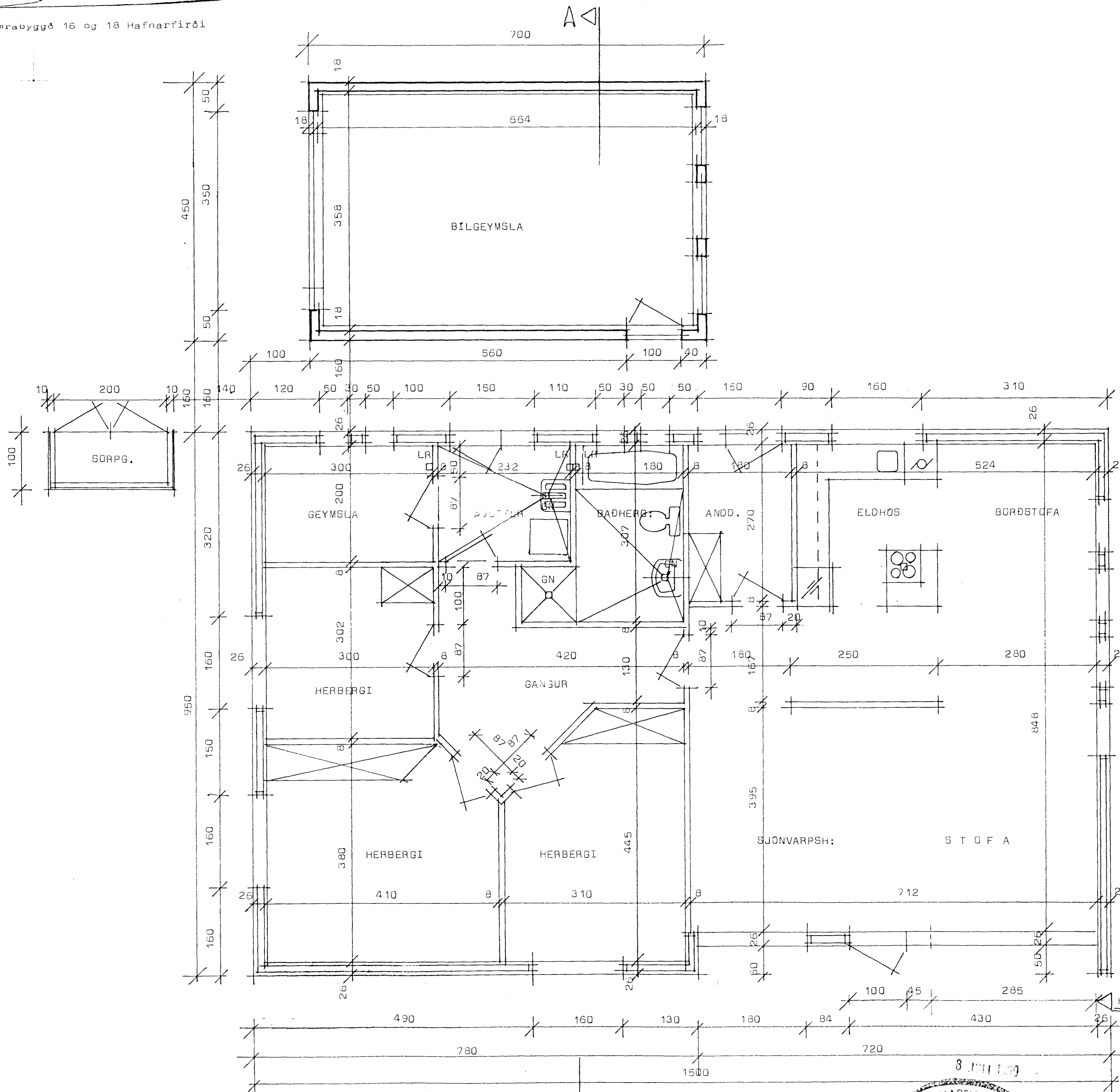
Grunnmynd Mk 1:50
