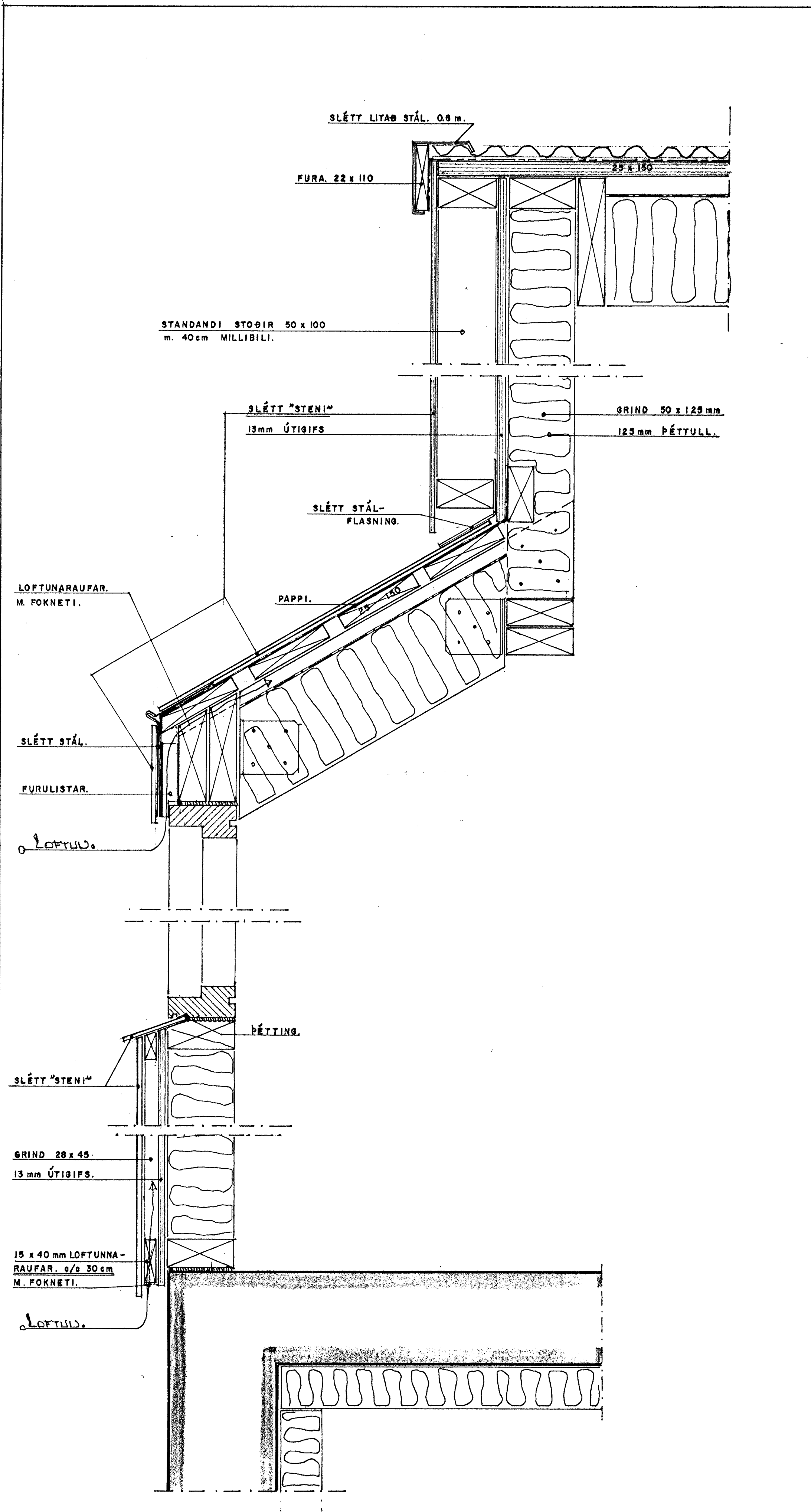
SNEIÐING GEGNUM ÚTBYGGINGU. 1:5
