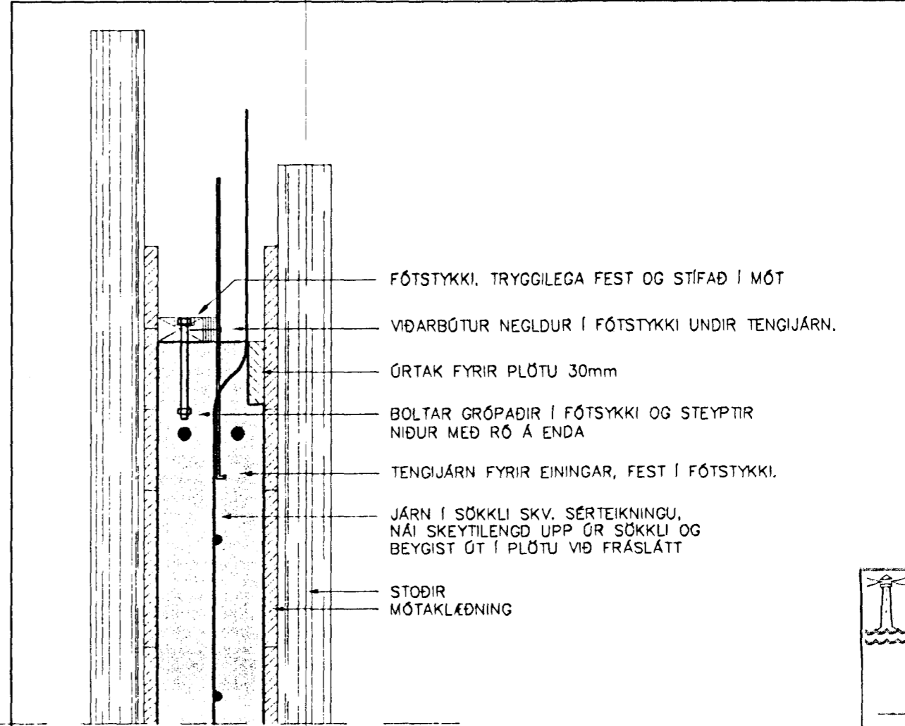
UPPSLÁTTUR Mkv. 1:10
