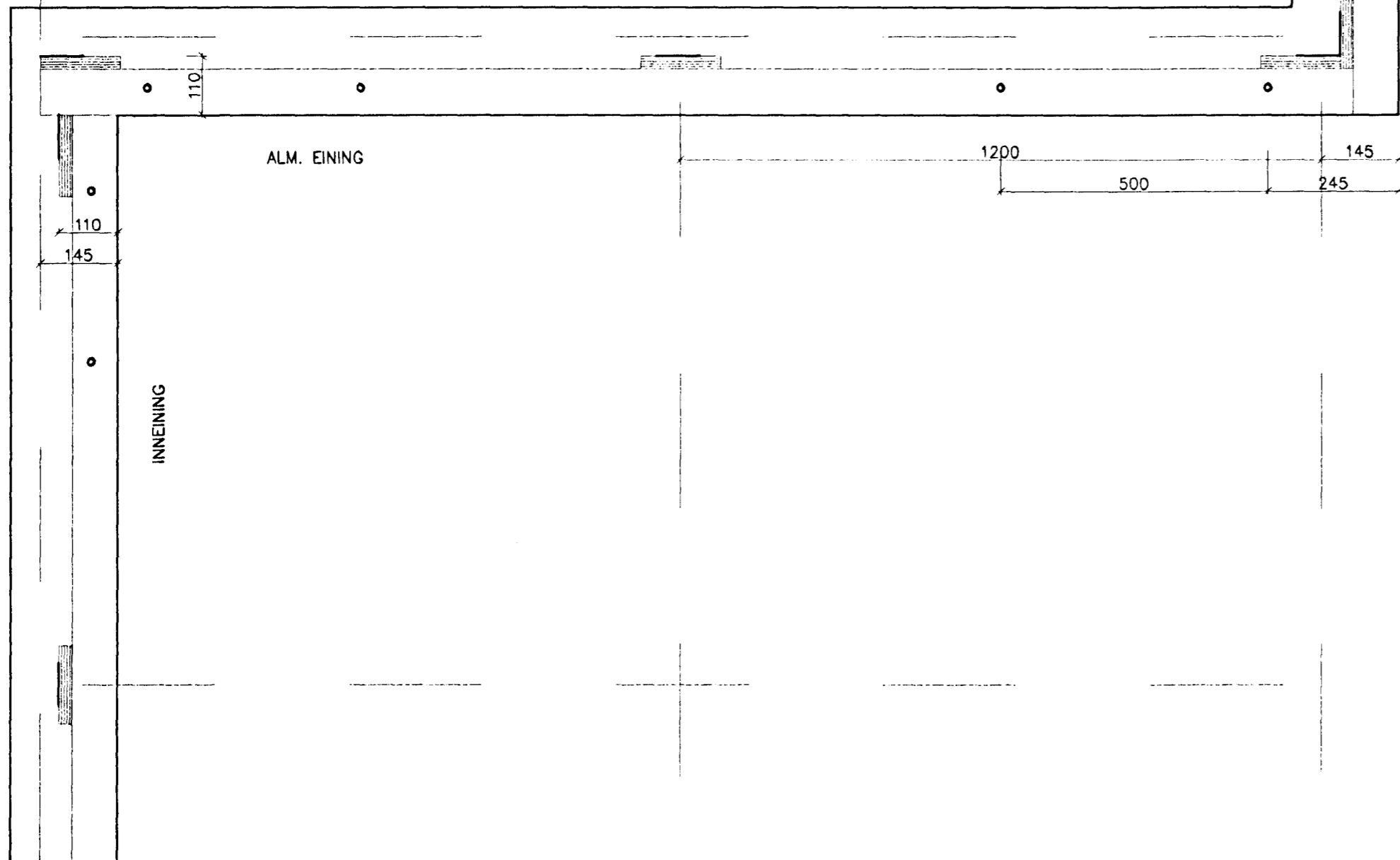
FRÁGANGUR FESTINGA Í SÖKKLI Mkv. 1:10
