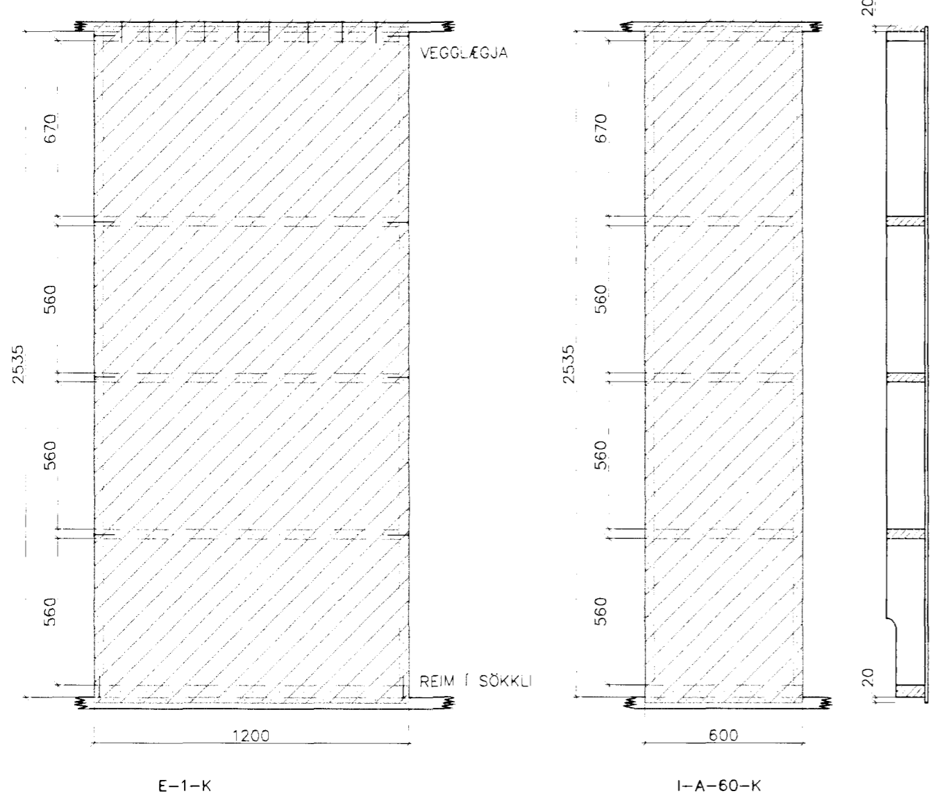
KROSSVIÐARSTÍFINGAR Mkv. 1:20
