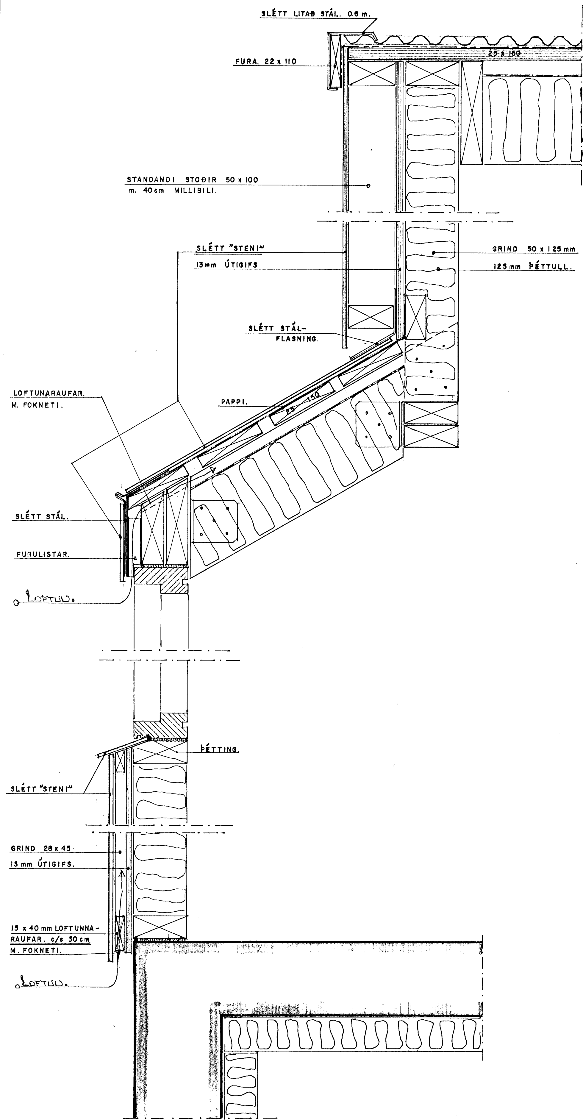
SNEIÐING GEGNUM ÚTBYGGINGU. 1:5
