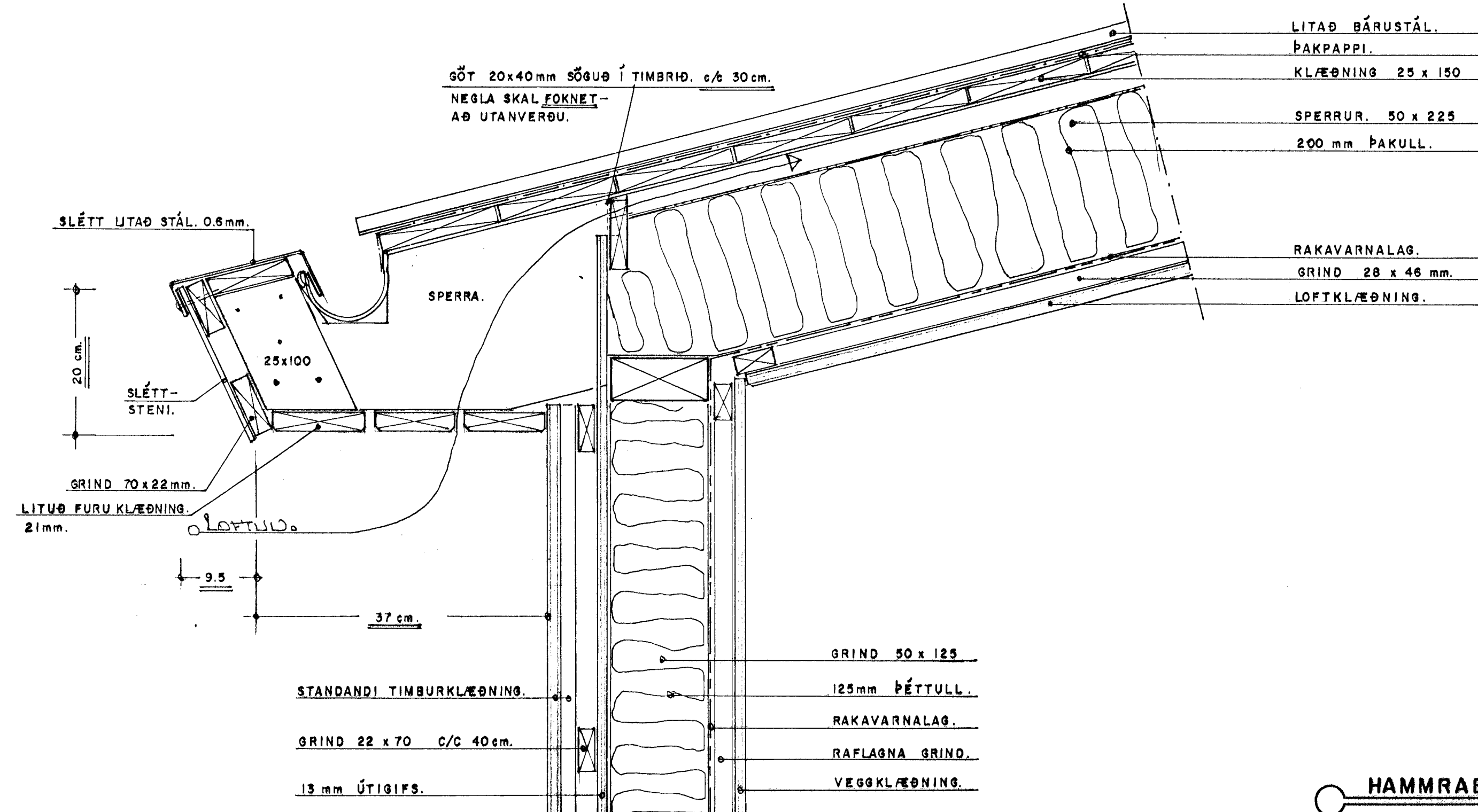
ÞAKKANTUR. 1:5
