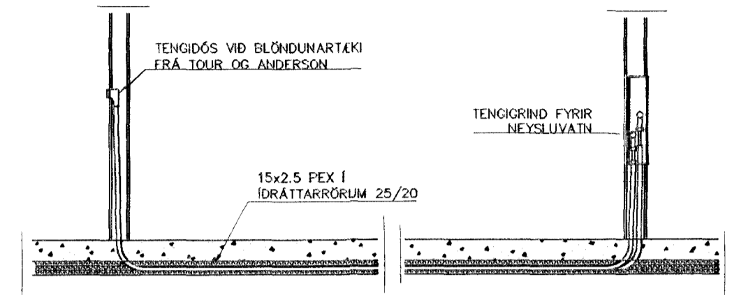
TENING NEYSLUVATNSLAGNA
