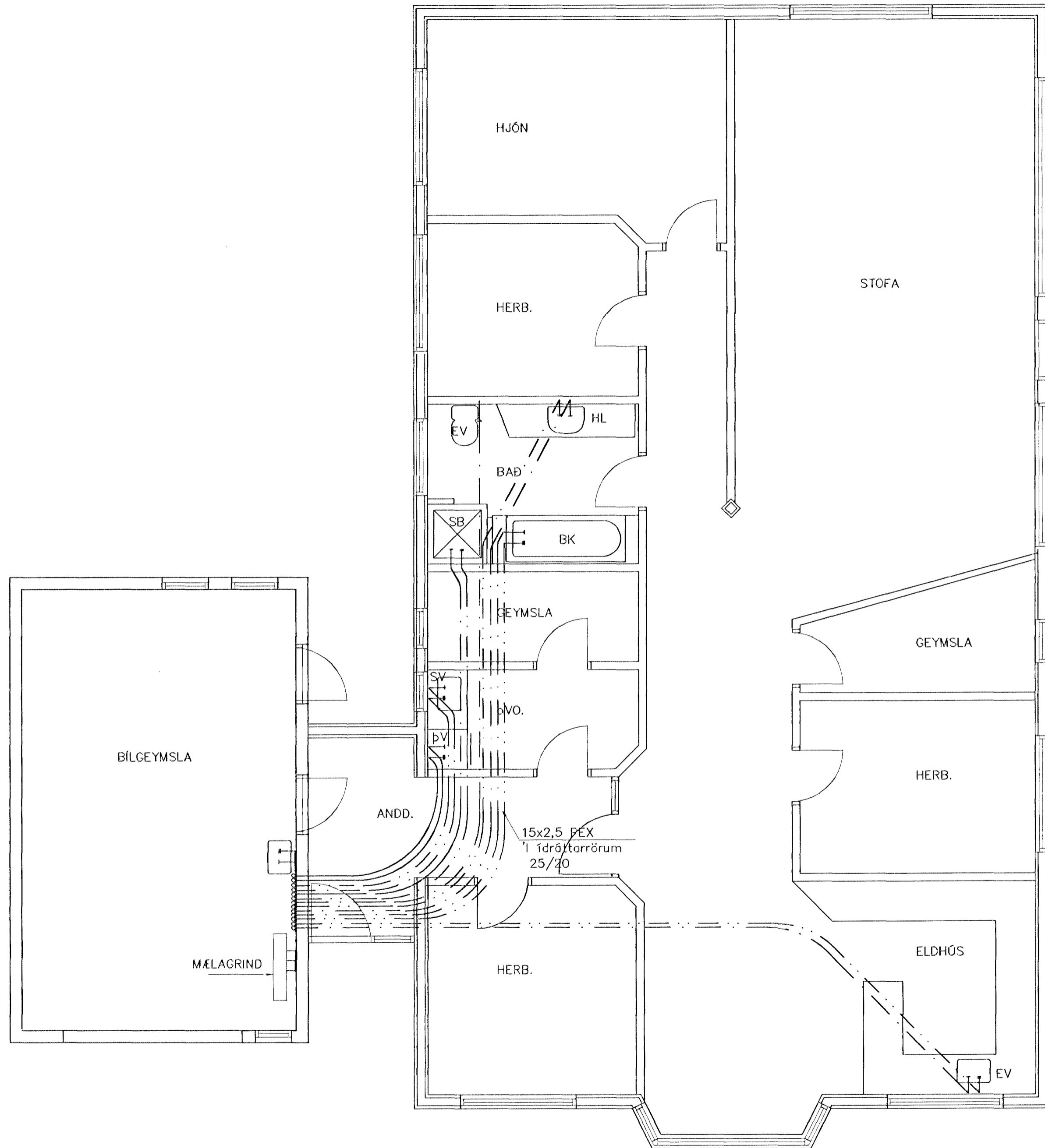
GRUNNMYND 1:50
