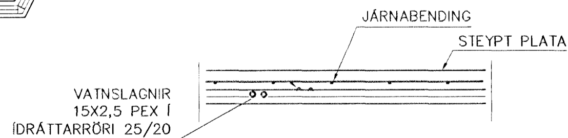
LAGNIR, SNIÐ, 1:20
