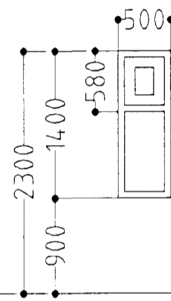
1 STK. ÞVÖTTUR. HURÐ OPNAST VINSTRI INN.
