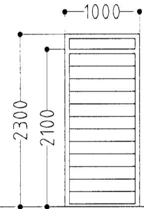
1 STK. BIFREIÐAGEYMSLA. HURÐ OPNAST HÆGRI ÚT.
