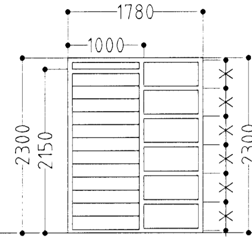
1 STK. ANDDYRI. HURÐ OPNAST VINSTRI ÚT.
