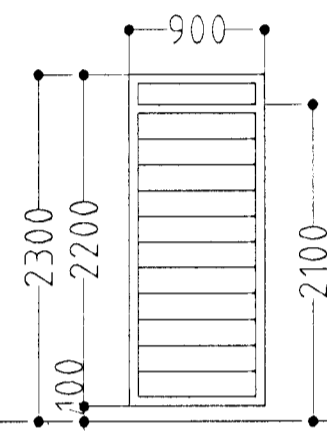
1 STK. ÞVÖTTUR. HURÐ OPNAST VINSTRI INN.
