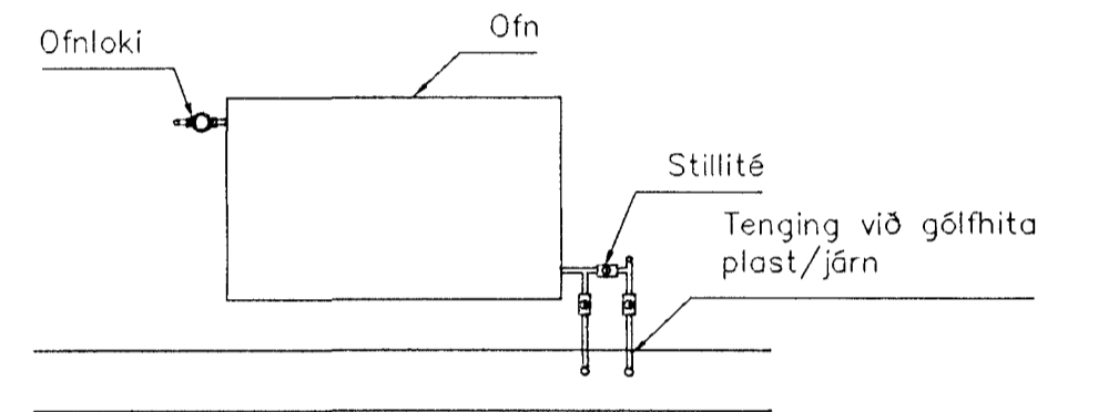
Tenging gólfhita
