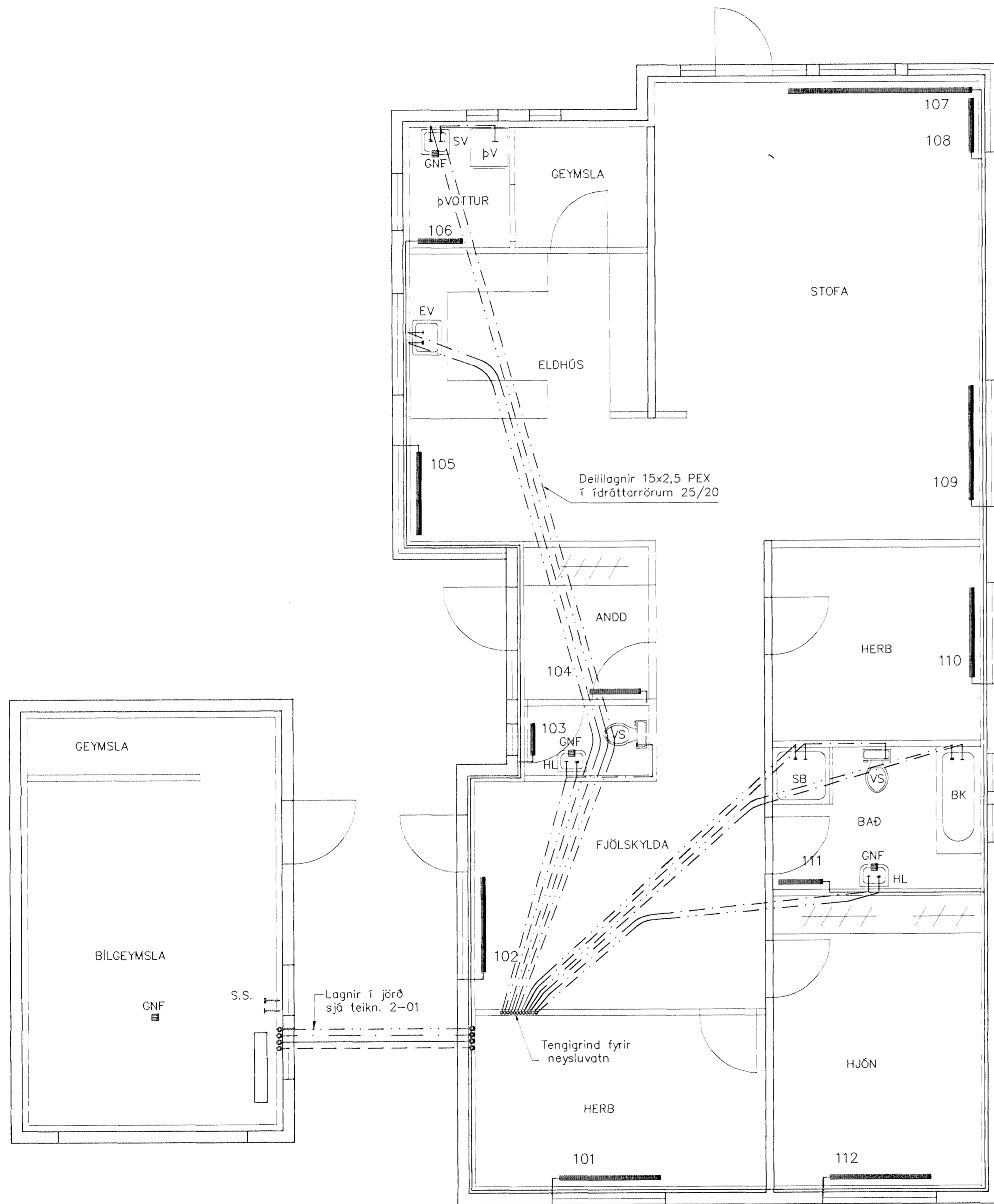
GRUNNMYND 1:50
