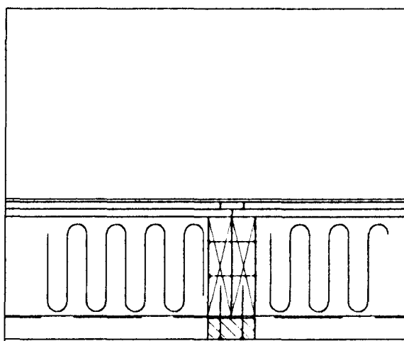
LÁRÉTT SNID Í VEGG Mkv. 1:10
