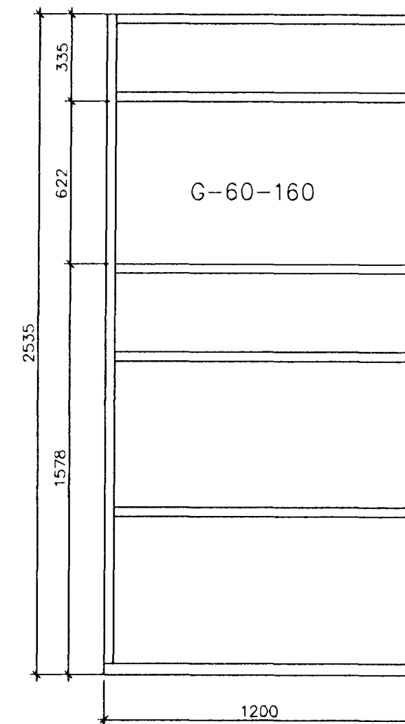
SKÝRINGARMYND FYRIR EININGAR Mkv. 1:20
