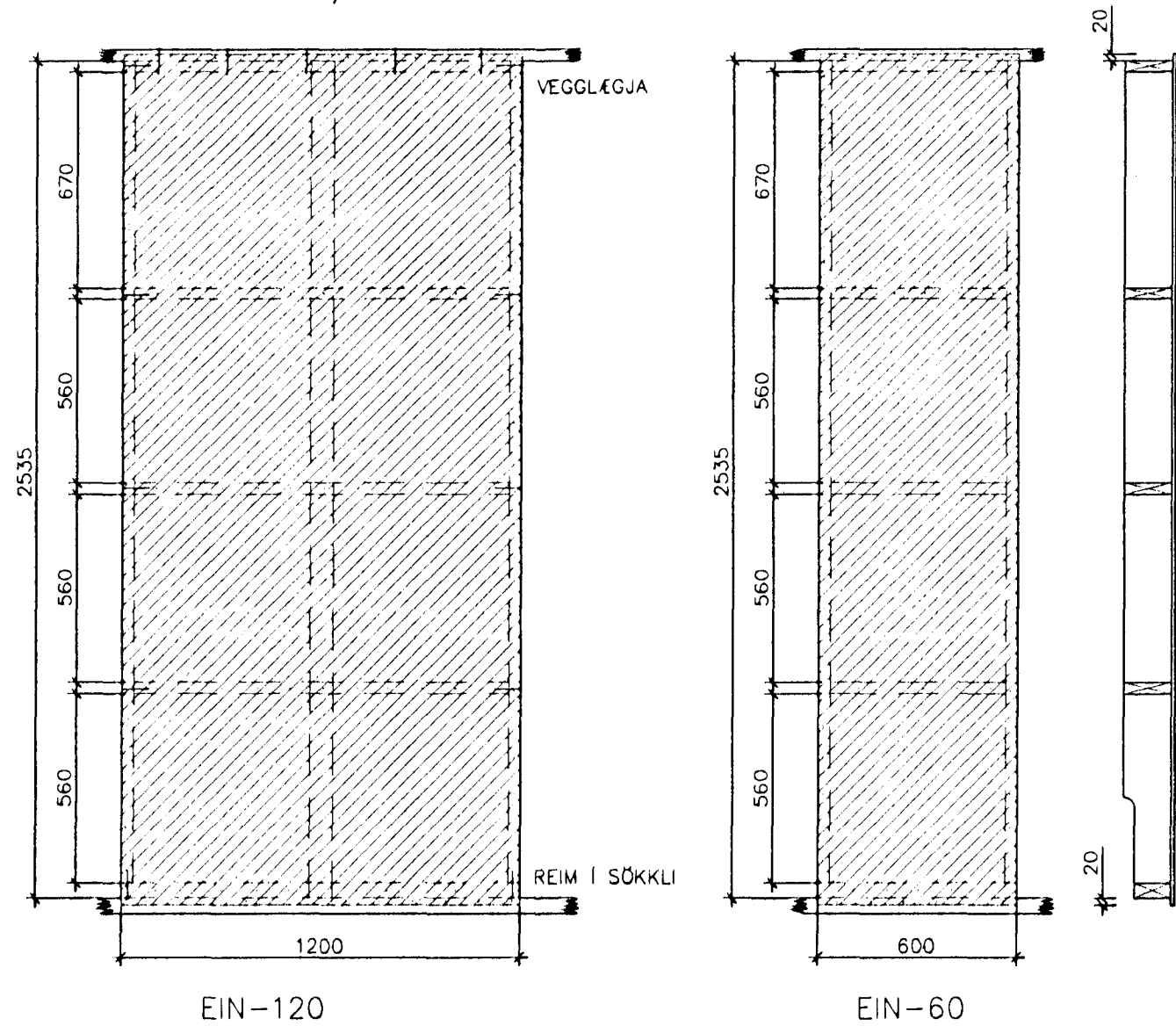
KROSSVÐARSTÍFINGAR Mkv. 1:20
