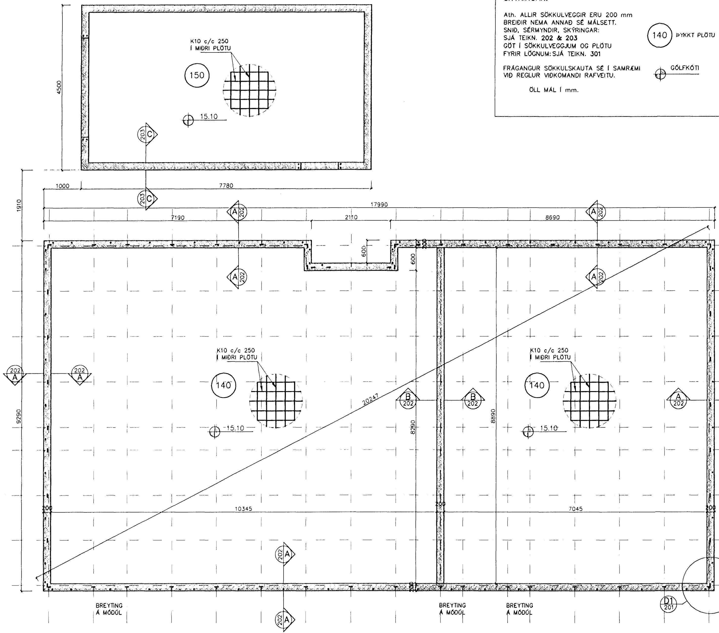
GRUNNMYND SÖKKULS Mkv. 1:50
