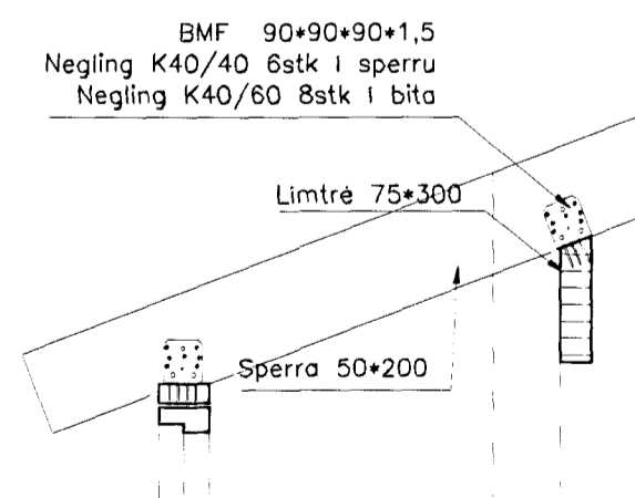
108 FESTING SPERRU VID BITA OG GLUGGASYLLU Mkv: 1/20
