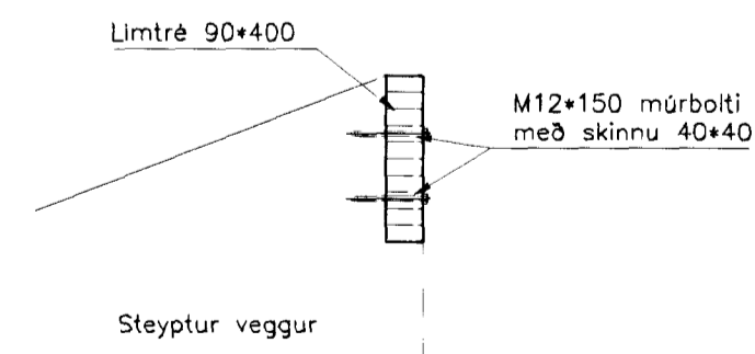
112 FESTING BITA VID STEYPTAN VEGG Mkv: 1/20
