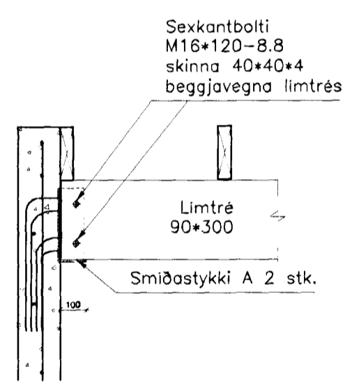
109 FESTING LÍMTRÉSBITA UNDIR SKYGGNI Mkv: 1/20
