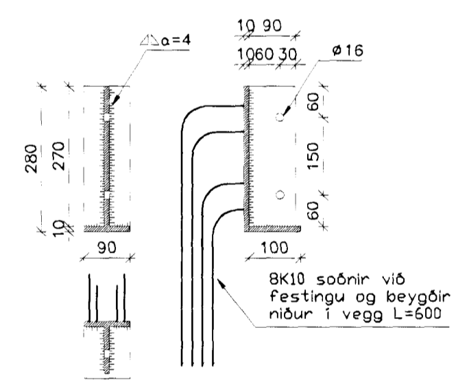
MÁLSETNING JÄRNFESTINGAR VID BITA Mkv: 1/10
