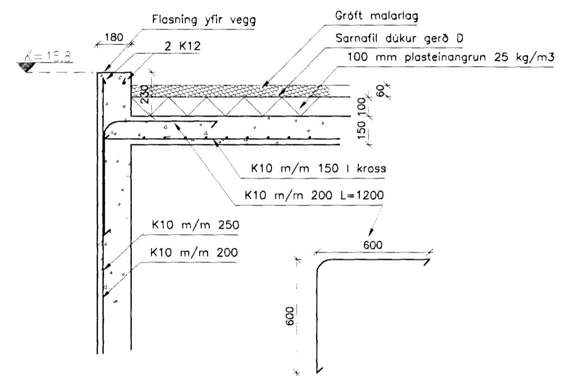
110 DEILI VID MÆNI Mkv: 1/20
