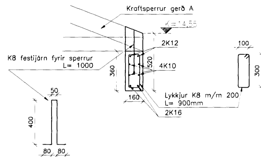
107 SKURDUR VID SYLLUSTYKKI Mkv: 1/20
