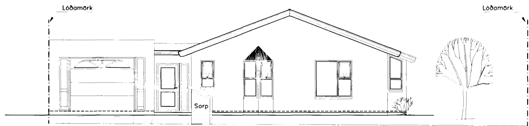
ÚTLIT NORDAUSTUR Mkv: 1/100
