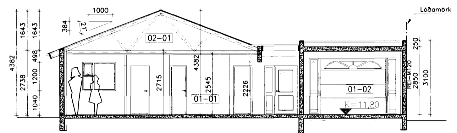
SKURÐUR C-C
