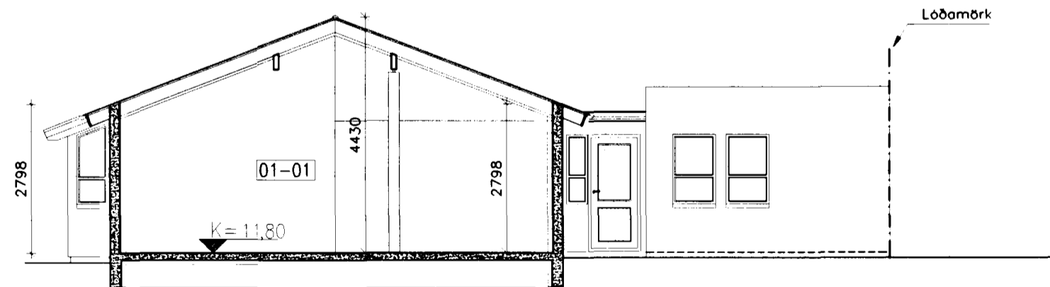
SKURÐUR A-A
