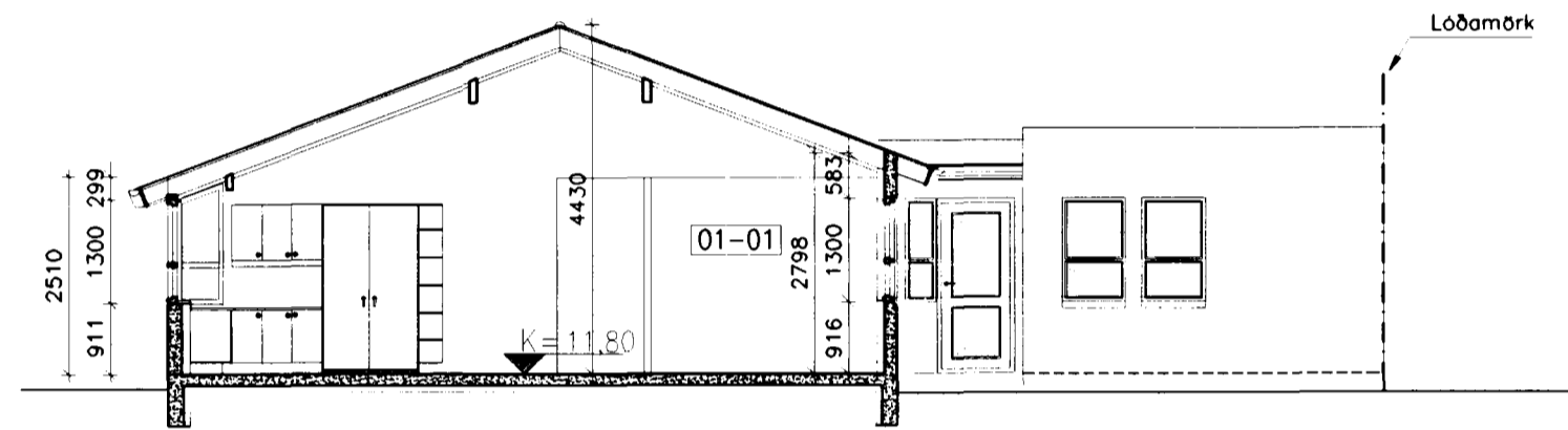
SKURÐUR B-B
