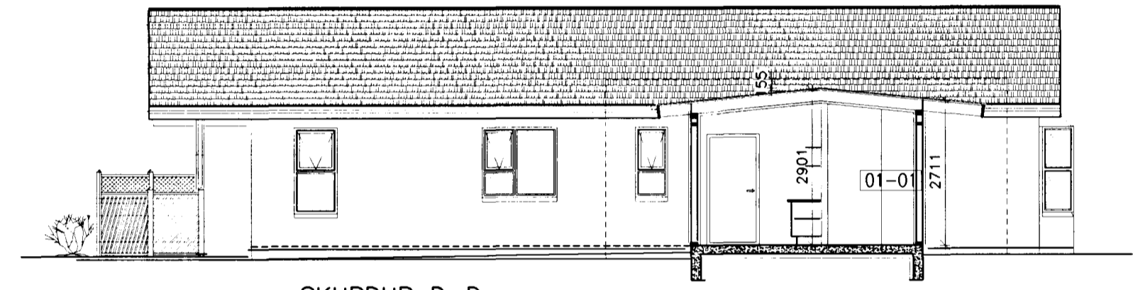
SKURÐUR D-D
