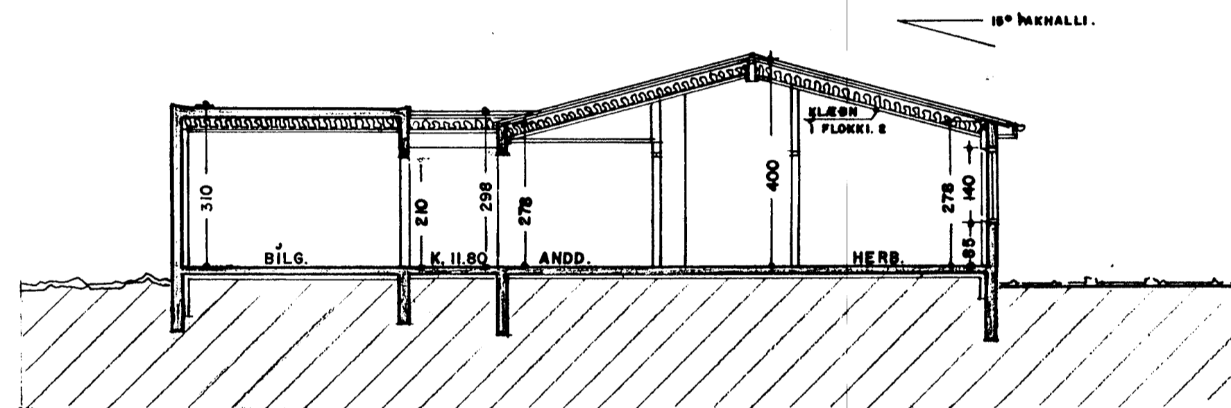
SNEIÐING 1:100
