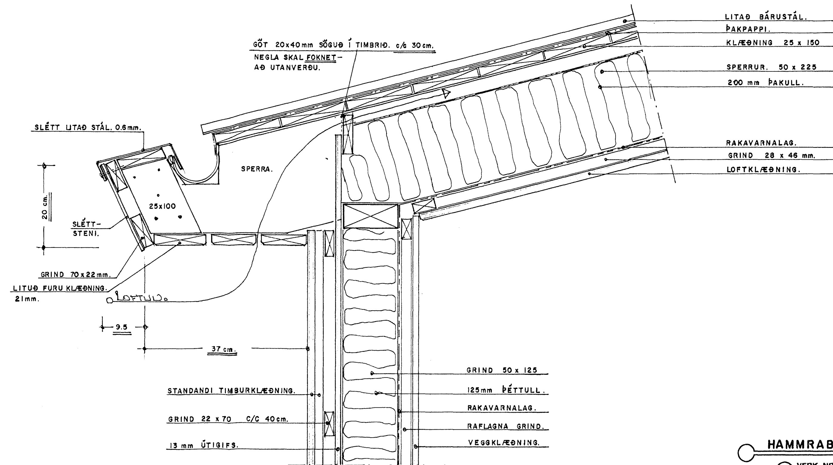
ÞAKKANTUR. 1:5
