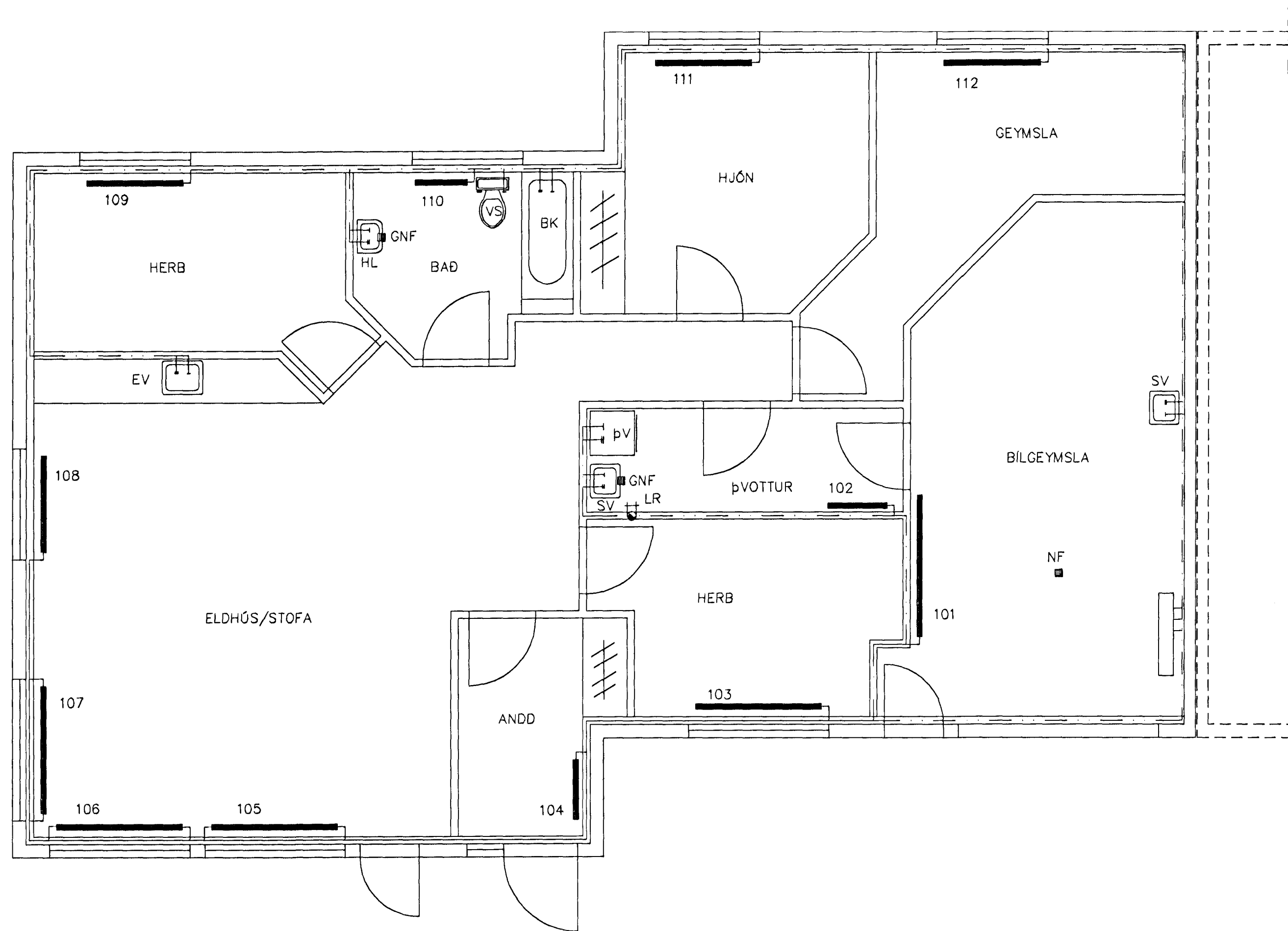
GRUNNMYND 1:50
