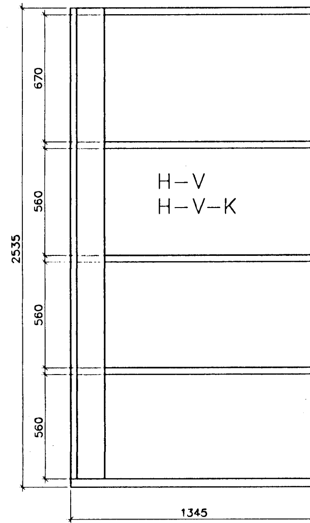
ÞVERSNIÐ Í HORNEININGAR
