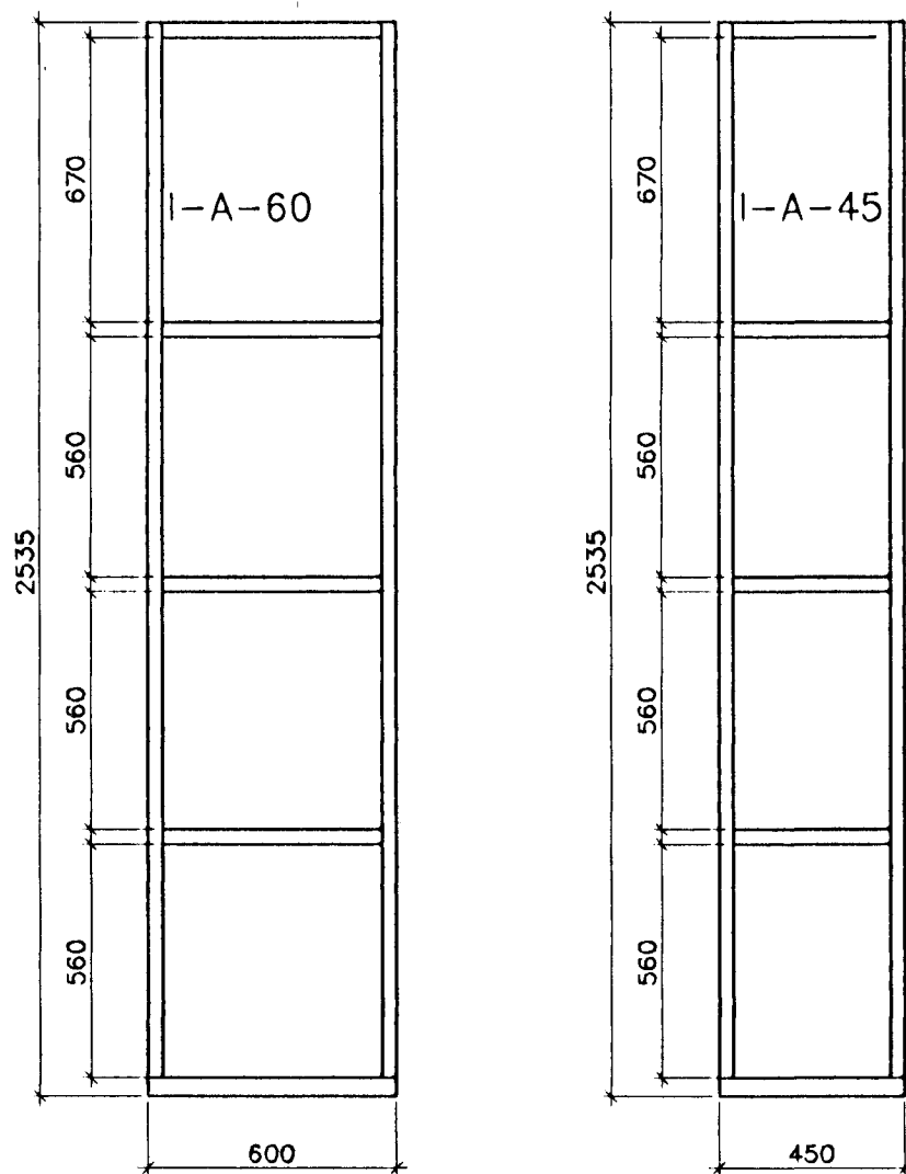
SKÝRINGARMYND FYRIR ENINGAR Mkv. 1:20
