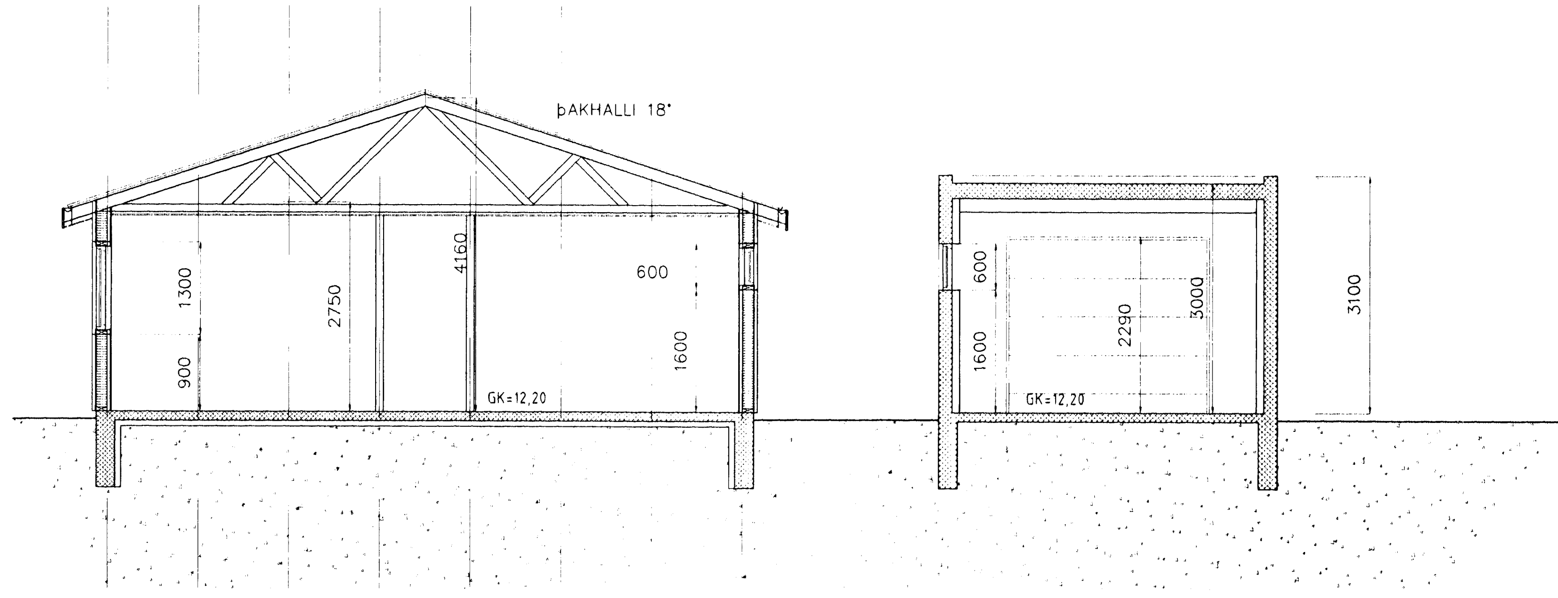
SNIÐ A-A
