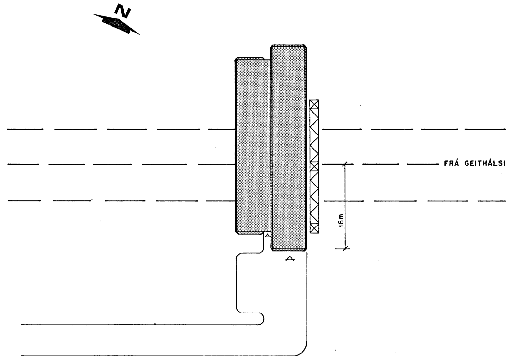
AFSTÖÐUMYND M=1:500
