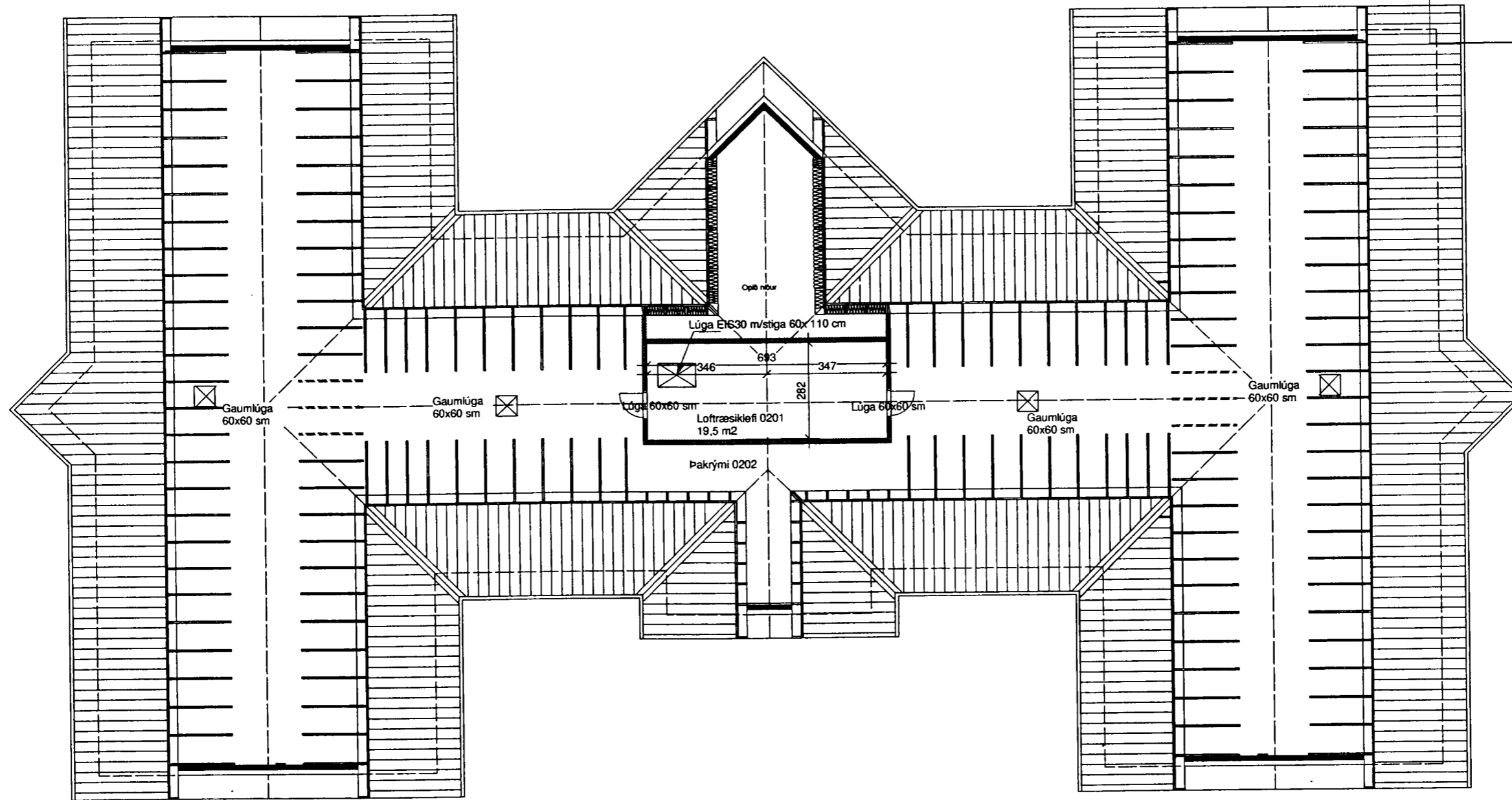
Grunnmynd þaks
