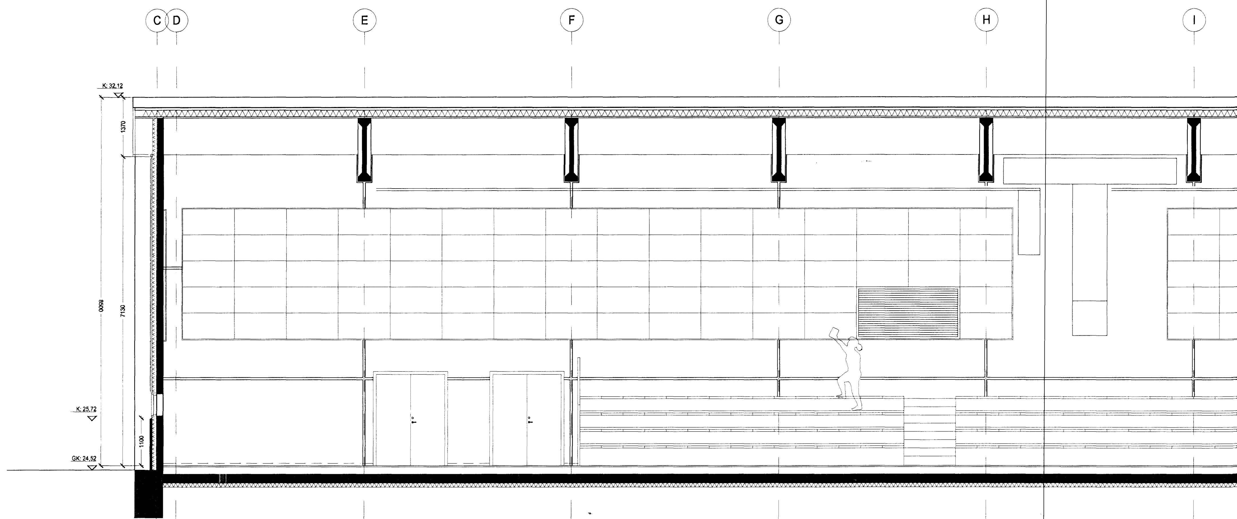
Sneiðing E-E
