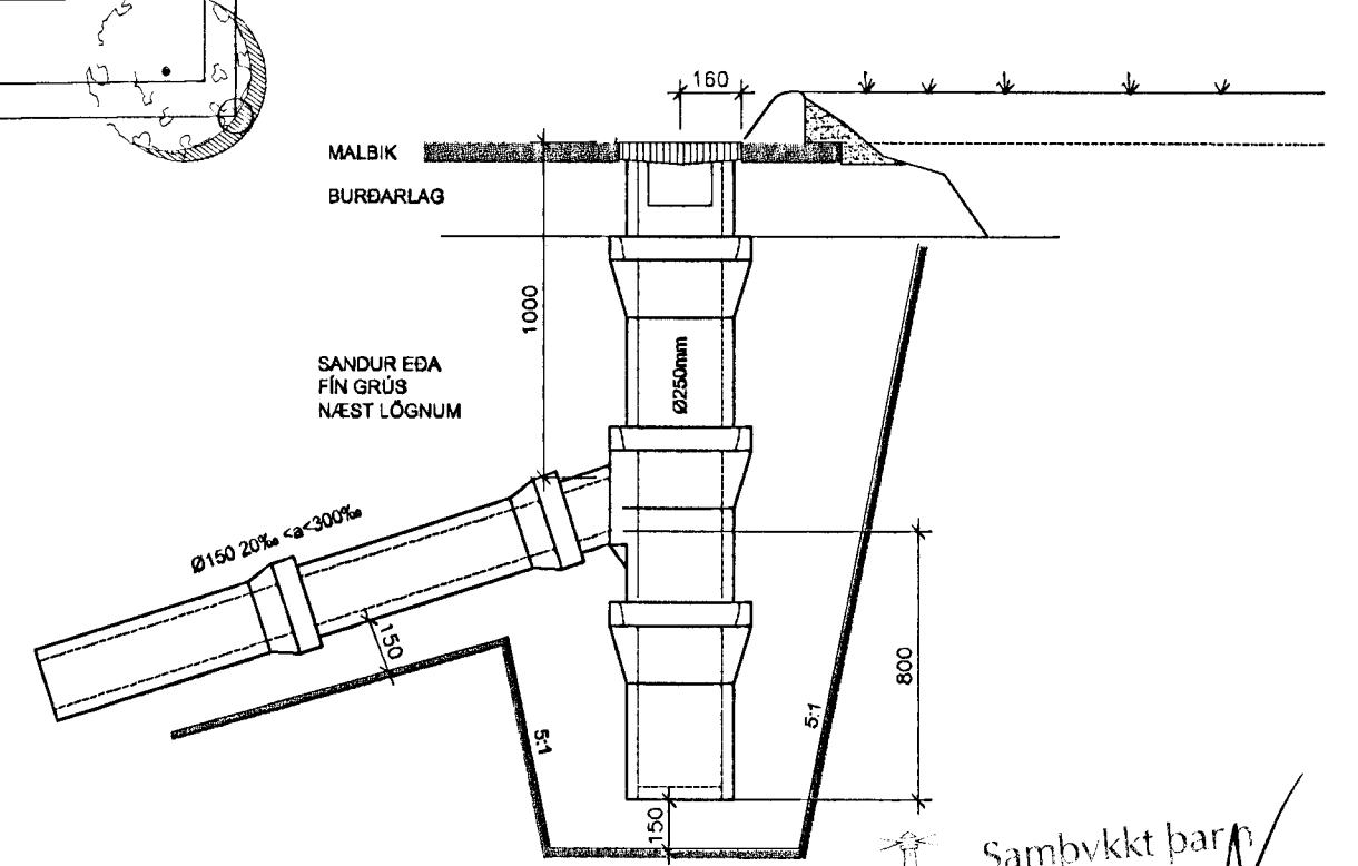
NÍÐURFALL 1:20
