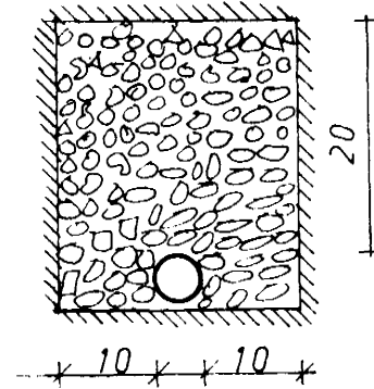
JARÐVATNSLÖGN ÞVERSNIÐ 1:10
