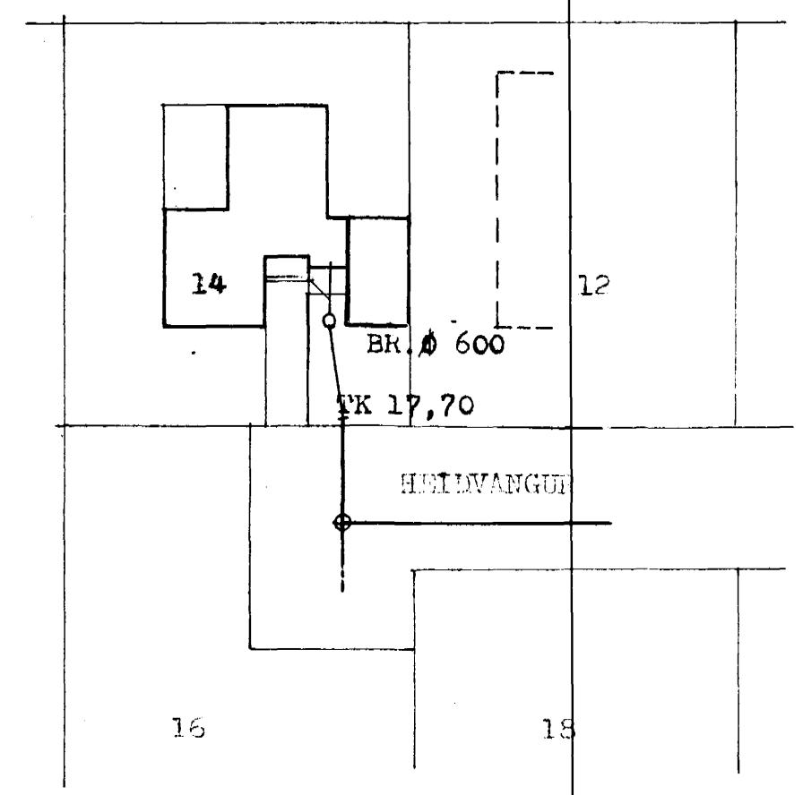
AFSTADA 1:500
