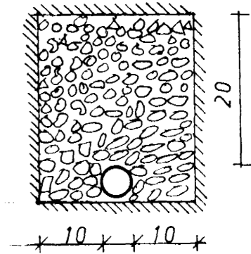
JARÐVATNSLÖGN ÞVERSNÍÐ 1:10
