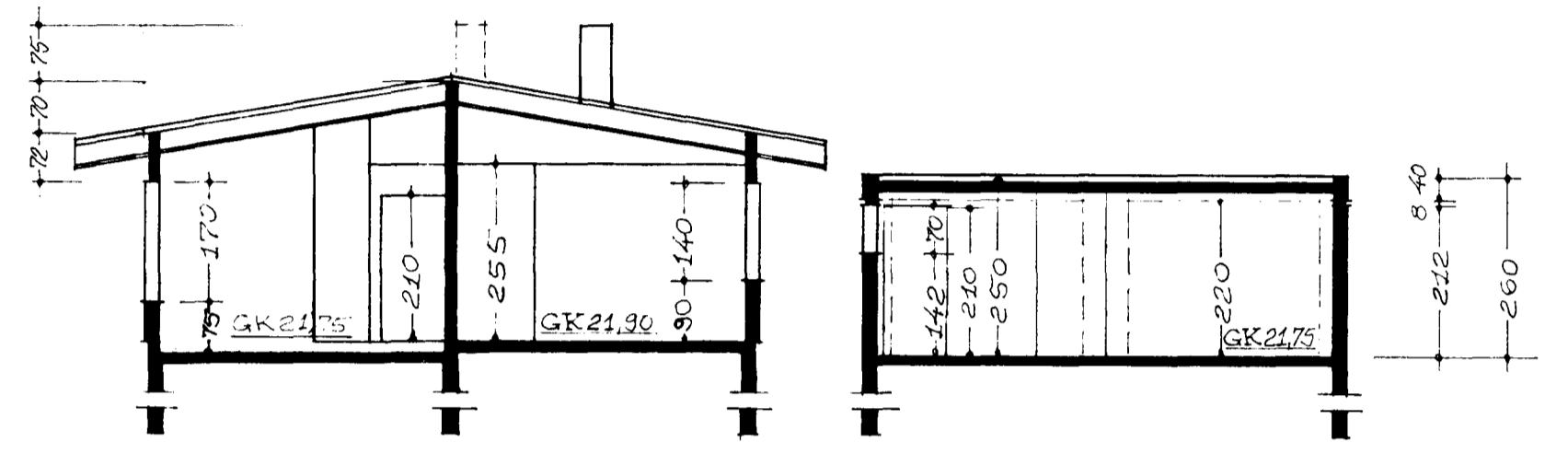
SKURÐUR A-A
