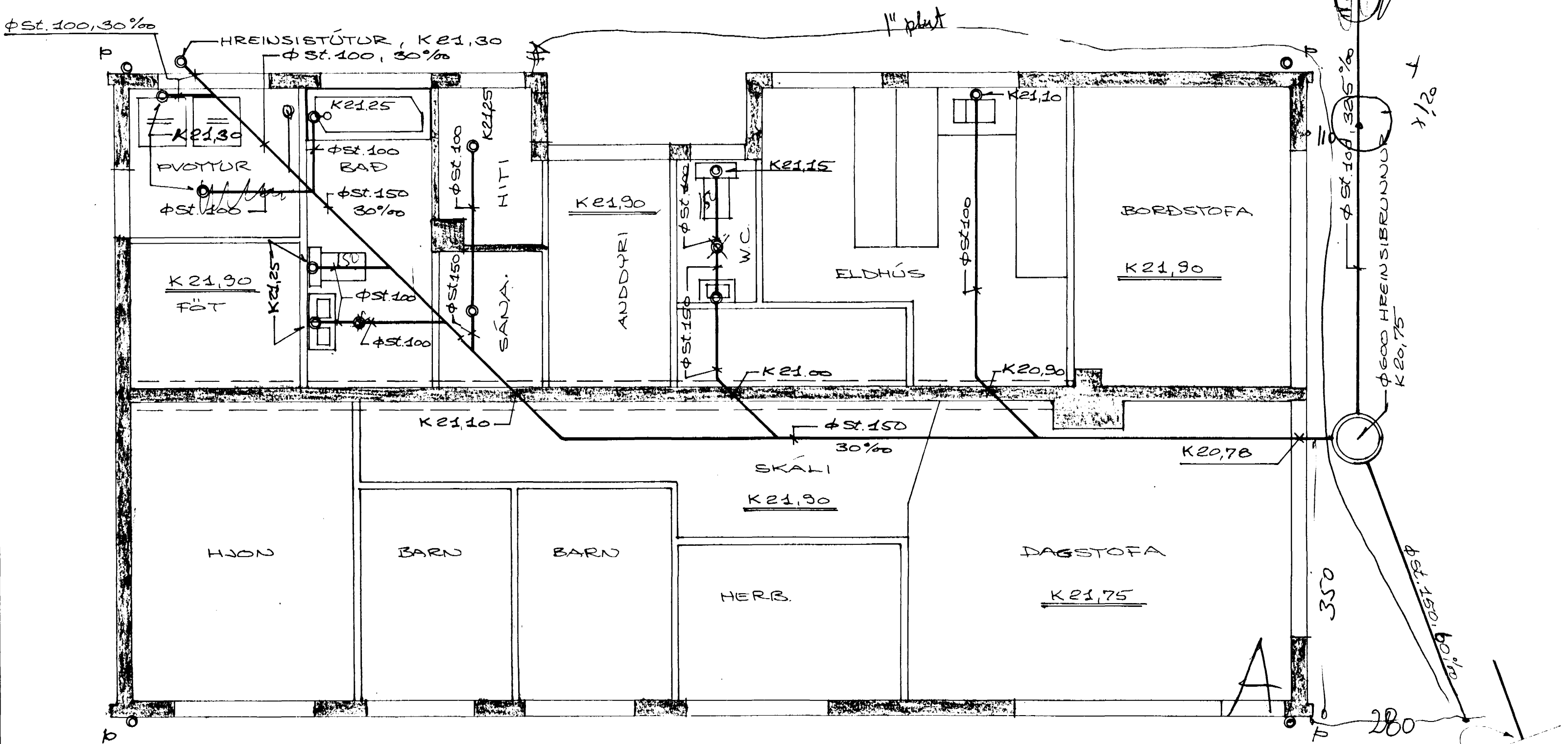
GRUNNMYND, M = 1:50
