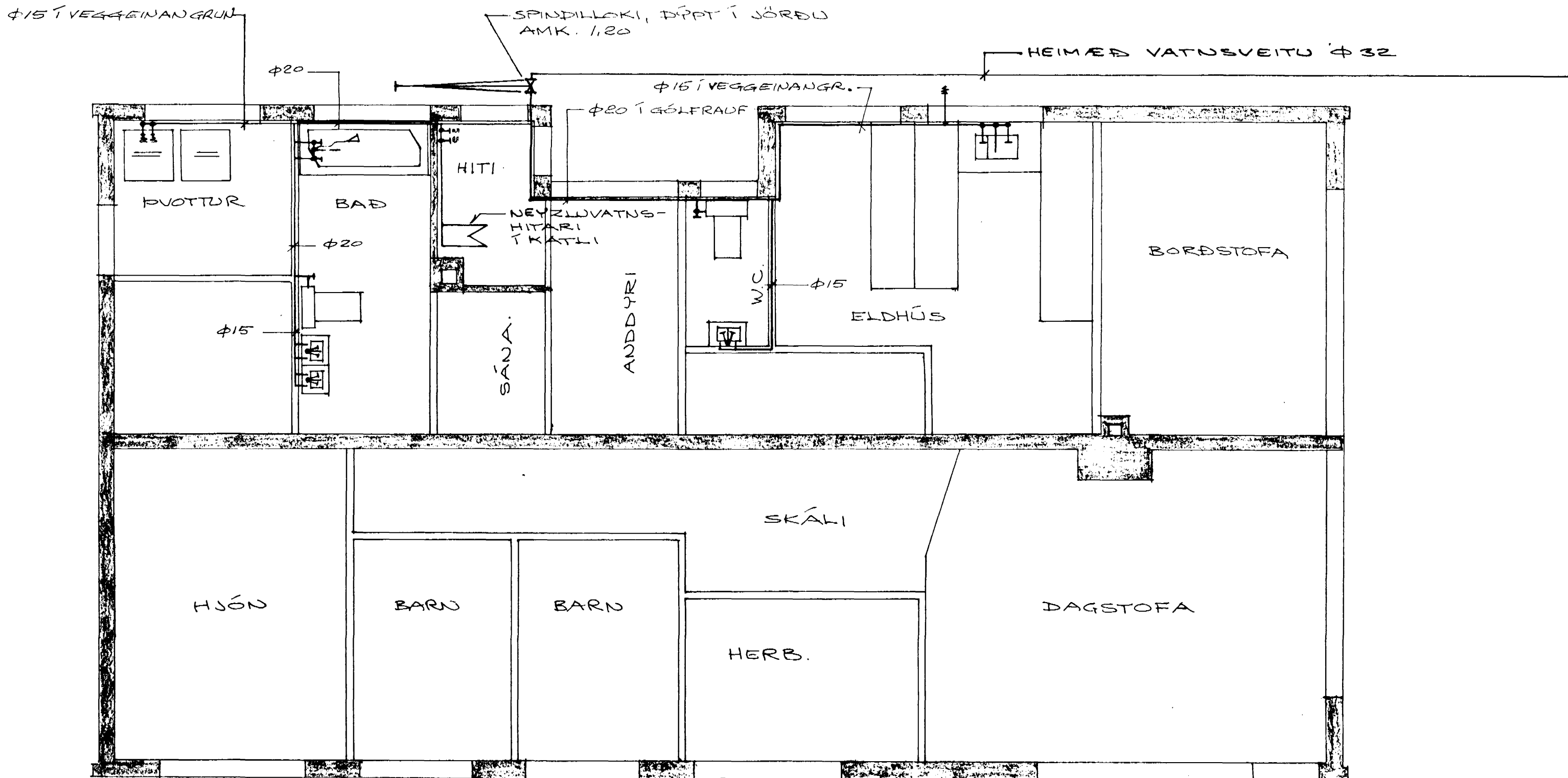
GRUNNMÝND, M = 1:50
