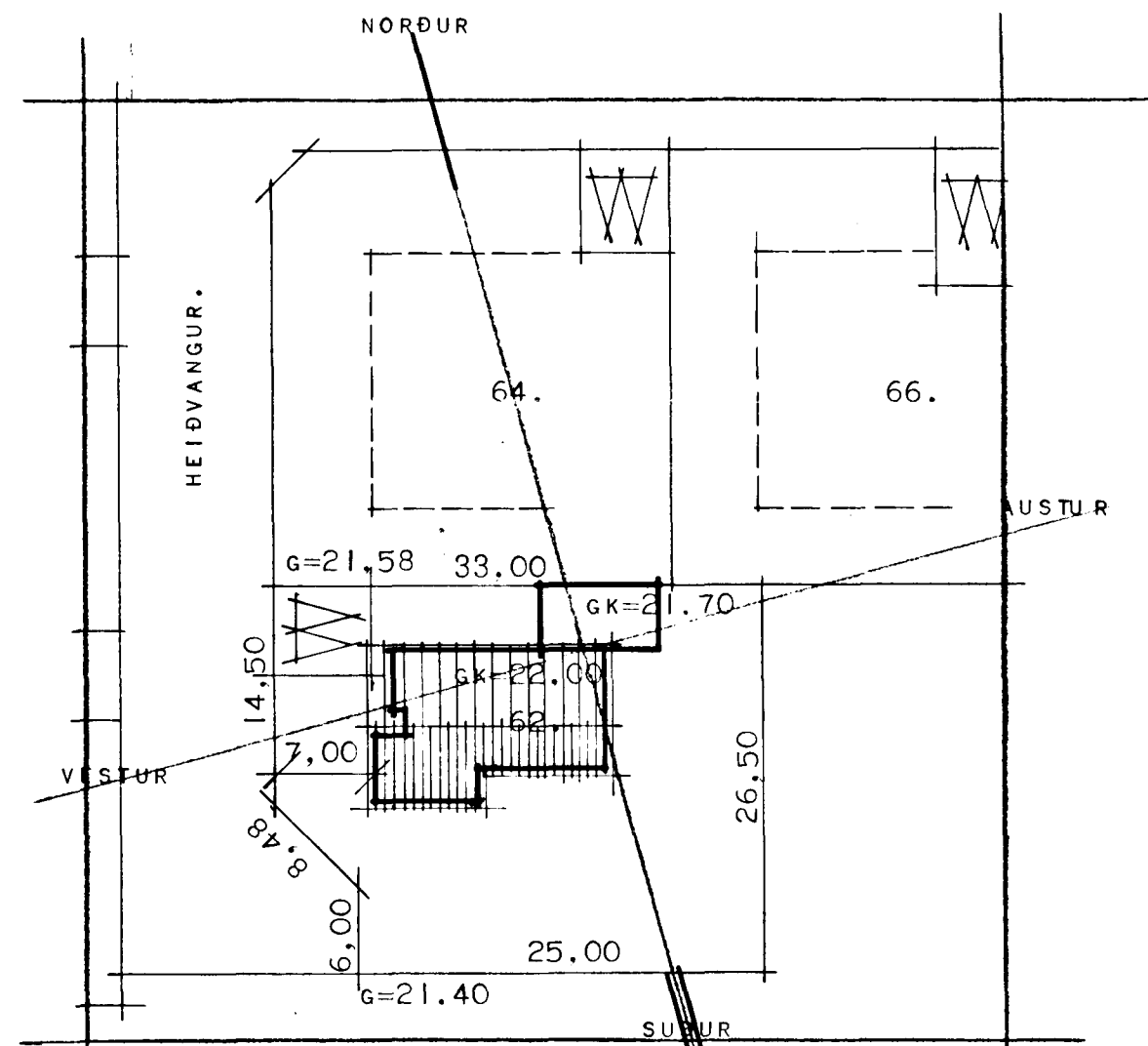
AFSTÖÐUMYND MÁL 1:500
