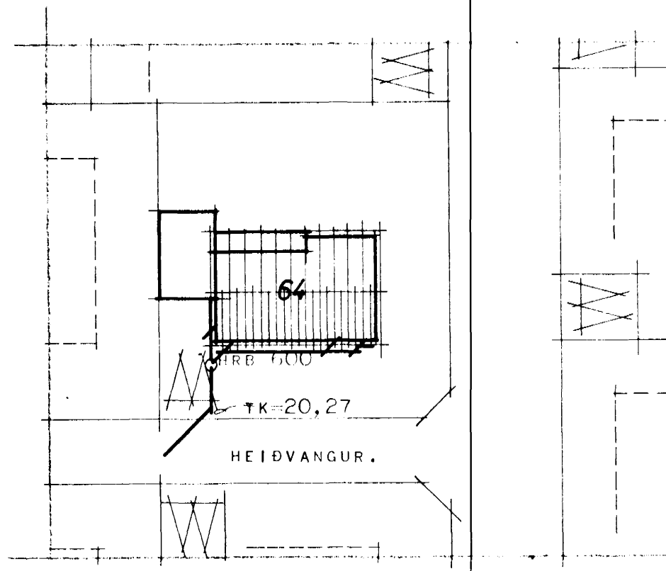
AFSTÖÐUMYND MÁL 1:500
