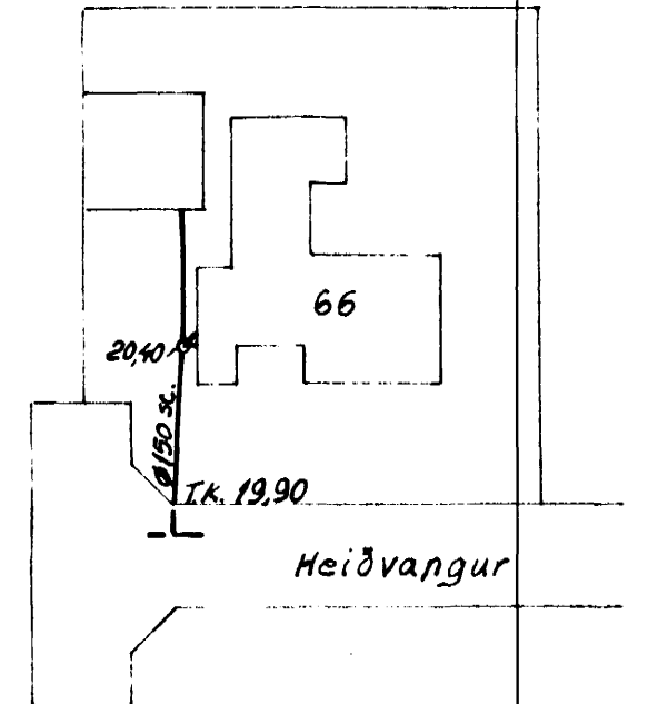
Afstöðumynd 1:500
